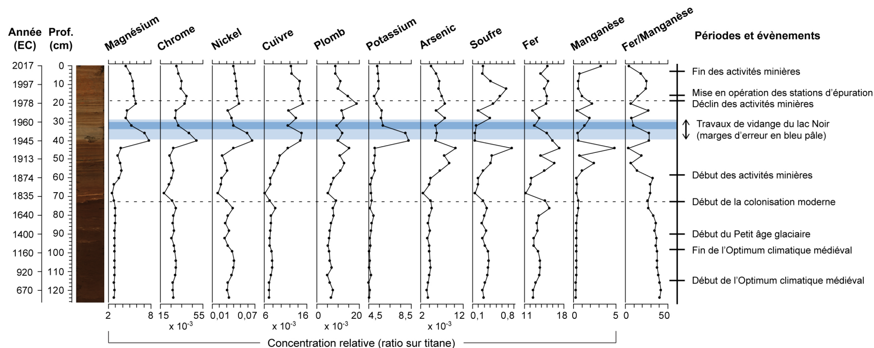
Figure 9.6. Profils de variation de la concentration relative (vis-à-vis le titane ou le manganèse) de certains métaux sélectionnés dans la carotte de sédiments du lac William. Note : les traits pointillés marquent le début de la colonisation moderne de la Haute-Bécancour (~ 1810 EC) et le début du déclin des activités minières d'amiante (1980 EC).
