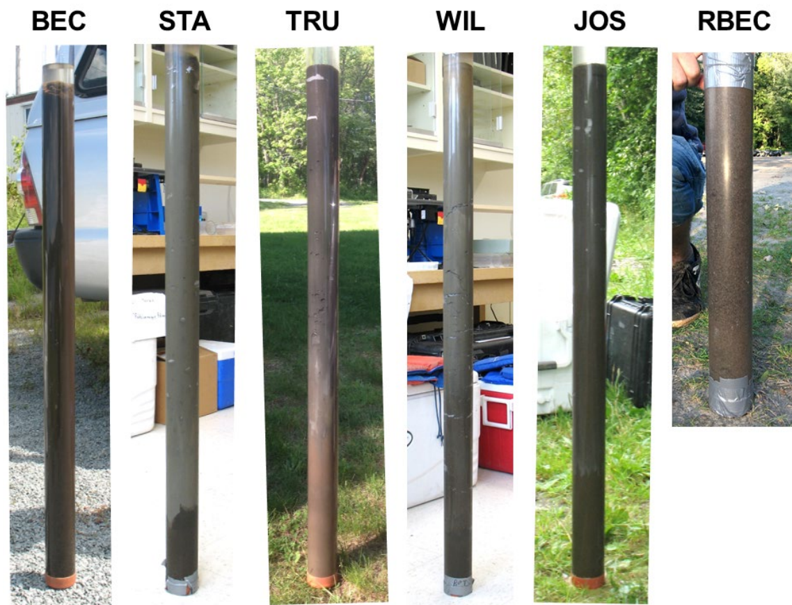
Figure 4.4. Photographies des carottes de sédiments prélevées dans le lac Bécancour (BEC), l'étang Stater (STA), le lac à la Truite (TRU), le lac William (WIL), le lac Joseph (JOS) et la rivière Bécancour (secteur du fleuve Saint-Laurent; RBEC), lesquelles font l'objet des analyses présentées dans ce rapport.
