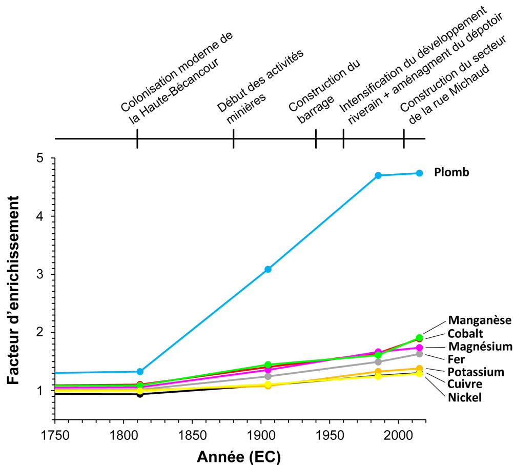
Figure 6.7. Évolution du facteur d'enrichissement de certains métaux sélectionnés dans les sédiments récents du lac Bécancour (1750–2017 EC). Note : les métaux présentés sont ceux ayant les facteurs les plus élevés depuis la colonisation moderne de la Haute-Bécancour (~ 1810 EC).
