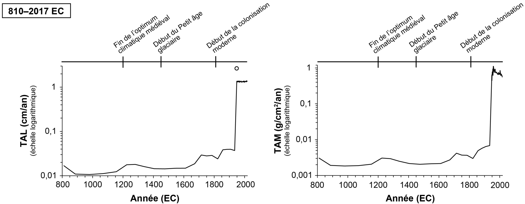
Figure 7.2. Évolution des taux d'accumulation linéaire (TAL; cm/an) et des taux d'accumulation massique (TAM; g/cm²/an) de sédiments à l'étang Stater. Note : les cercles vides désignent des valeurs aberrantes qui ont été exclues.
