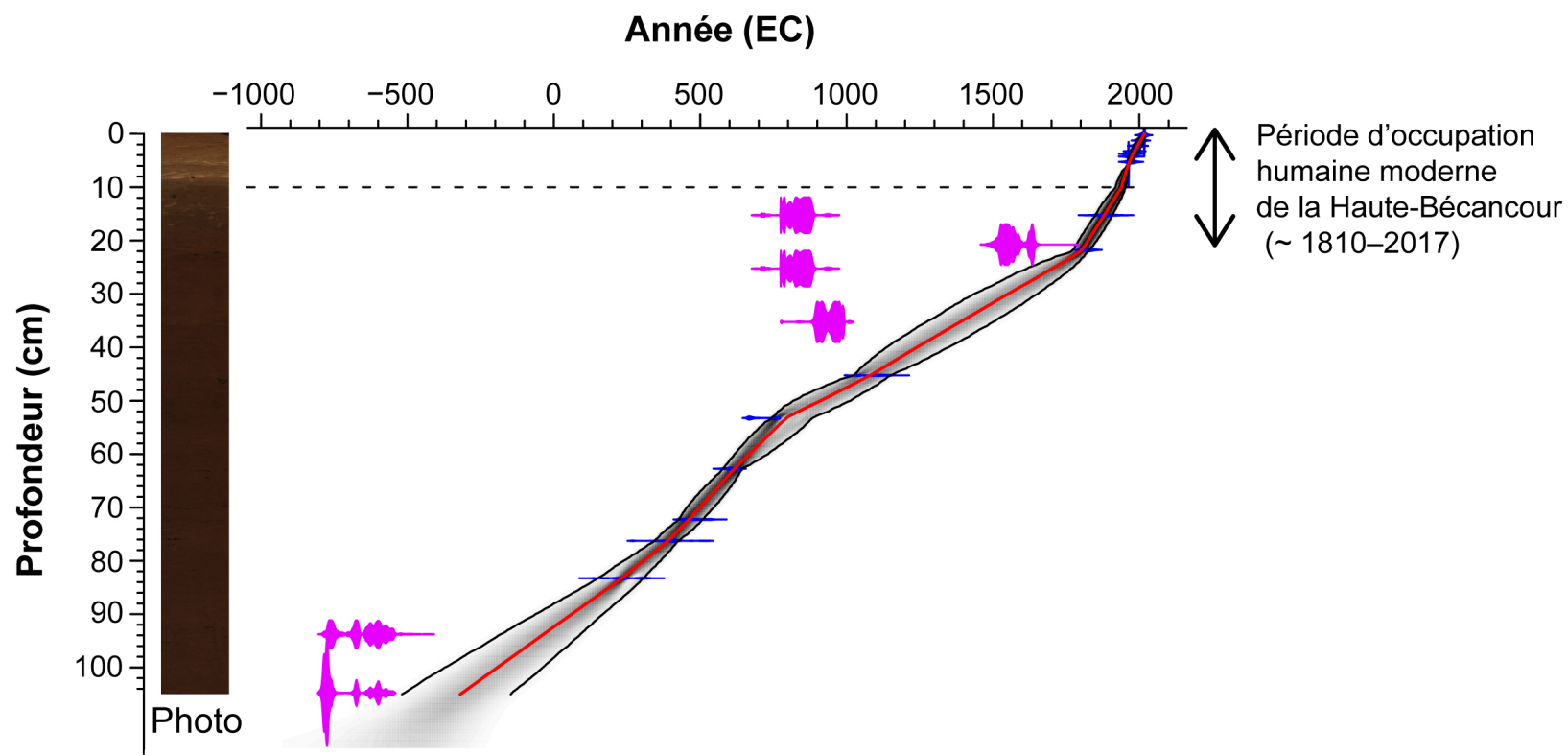
Figure 10.1. Présentation de la carotte de sédiments du lac Joseph et de son modèle chronologique. Note : la photo illustre l'intérieur de la carotte (plan longitudinal). La ligne rouge représente la courbe d'âge associée aux différents niveaux de profondeurs. Les lignes noires délimitent les intervalles d'erreur (niveau de confiance de 95 %). Les marqueurs bleus désignent les dates qui ont été retenues afin d'établir le modèle, tandis que les marqueurs mauves représentent les dates qui ont été exclues. La ligne pointillée horizontale délimite une coupure stratigraphique importante qui a été considérée dans l'élaboration du modèle chronologique.
