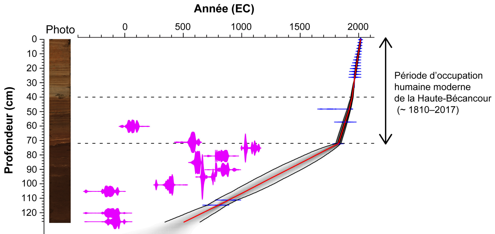
Figure 9.1. Présentation de la carotte de sédiments du lac William et de son modèle chronologique. Note : la photo illustre l'intérieur de la carotte (plan longitudinal). La ligne rouge représente la courbe d'âge associée aux différents niveaux de profondeurs. Les lignes noires délimitent les intervalles d'erreur (niveau de confiance de 95 %). Les marqueurs bleus désignent les dates qui ont été retenues afin d'établir le modèle, tandis que les marqueurs mauves représentent des dates qui ont été exclues. Les lignes pointillées horizontales délimitent des coupures stratigraphiques importantes qui ont été considérées dans l'élaboration du modèle chronologique.
