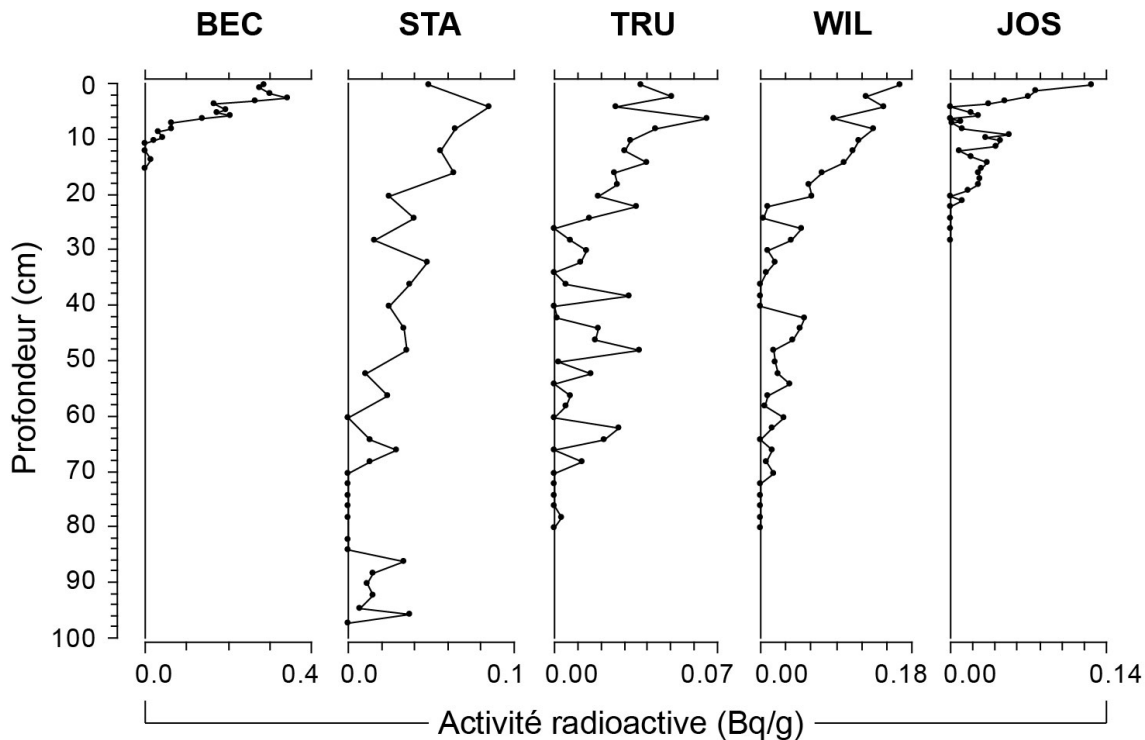
Figure 4.7. Profils de variation de l'activité radioactive du plomb 210 ( ^{210}\text{Pb} ) non supporté dans les carottes de sédiments du lac Bécancour (BEC), de l'étang Stater (STA), du lac à la Truite (TRU), du lac William (WIL) et du lac Joseph (JOS).
