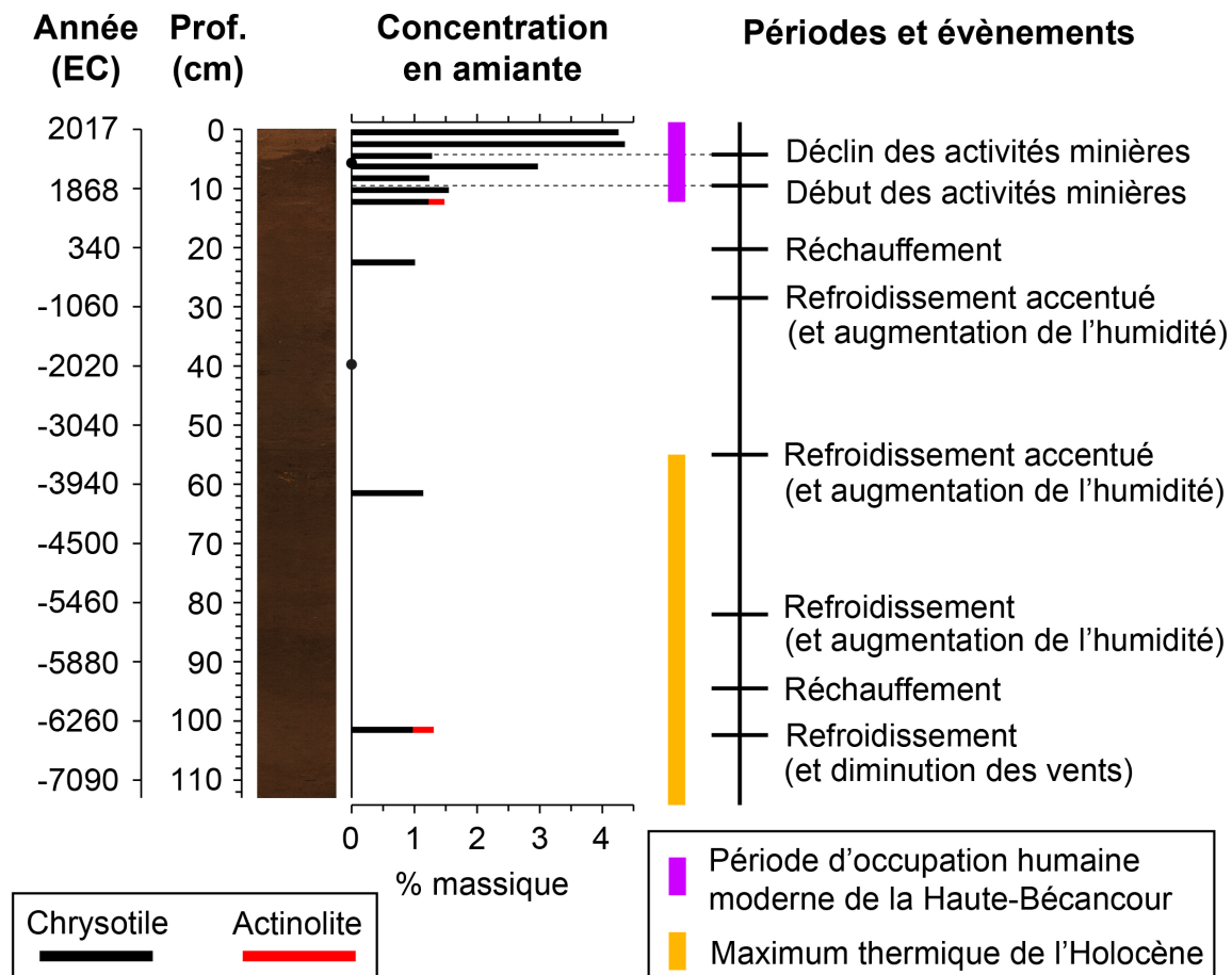
Figure 6.9. Concentration en fibres d'amiante à différents niveaux de profondeur de la carotte de sédiments du lac Bécancour. Note : les traits pointillés marquent le début des activités minières d'amiante dans la Haute-Bécancour (~ 1880 EC) et le début du déclin de l'industrie minière régionale (1980 EC).
