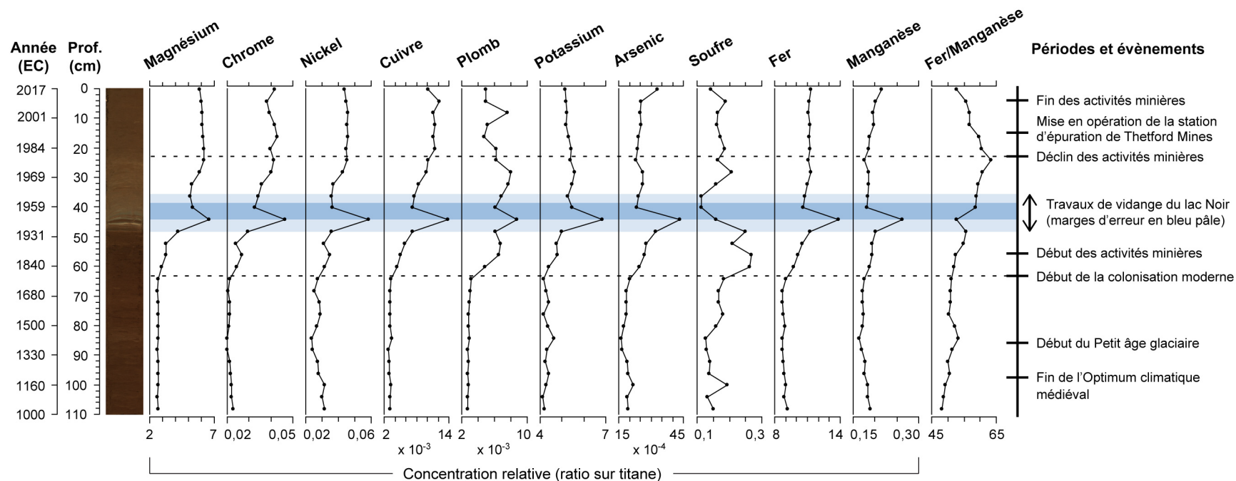
Figure 8.6. Profils de variation de la concentration relative (vis-à-vis le titane ou le manganèse) de certains métaux sélectionnés dans la carotte de sédiments du lac à la Truite. Note : les traits pointillés marquent le début de la colonisation moderne de la Haute-Bécancour (~ 1810 EC) et le début du déclin des activités minières d'amiante (1980 EC).
