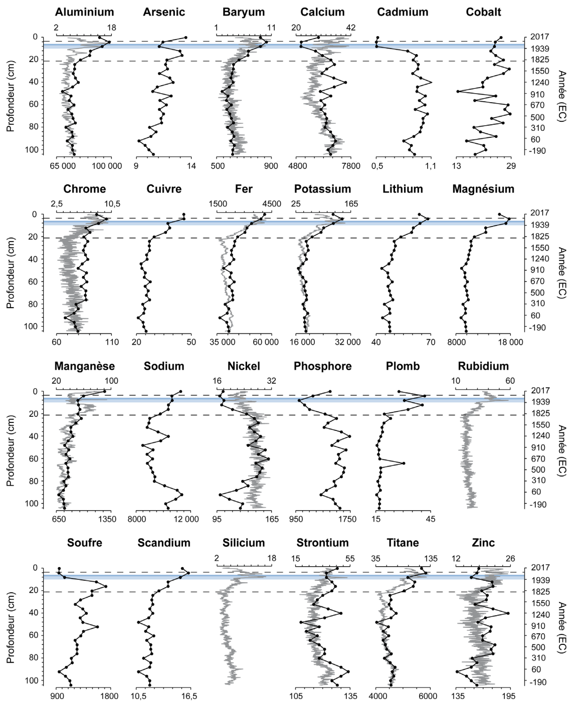
Figure 10.5. Profils de variation de la concentration absolue en métaux et autres éléments chimiques dans la carotte de sédiments du lac Joseph. Note : les courbes et points noirs (axes horizontaux inférieurs) représentent les données de concentrations (en mg/kg) établies par spectrométrie, tandis que les courbes grises (axes horizontaux supérieurs) correspondent aux données de concentrations relatives obtenues par microfluorescence X. Les zones colorées délimitent la période de travaux de vidange du lac Noir (1954–1959 EC; marges d’erreur en bleu pâle), tandis que les traits pointillés inférieur et supérieur marquent respectivement le début de la colonisation moderne de la Haute-Bécancour (~ 1810 EC) et le début du déclin des activités minières d’amiante (1980 EC).
