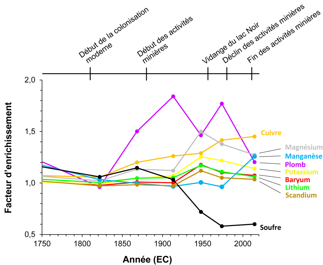
Figure 10.7. Évolution du facteur d'enrichissement de certains métaux sélectionnés dans les sédiments récents du lac Joseph (1750–2017 EC). Note : les métaux présentés sont ceux ayant les facteurs les plus élevés depuis la colonisation moderne de la Haute-Béancour (~ 1810 EC).
