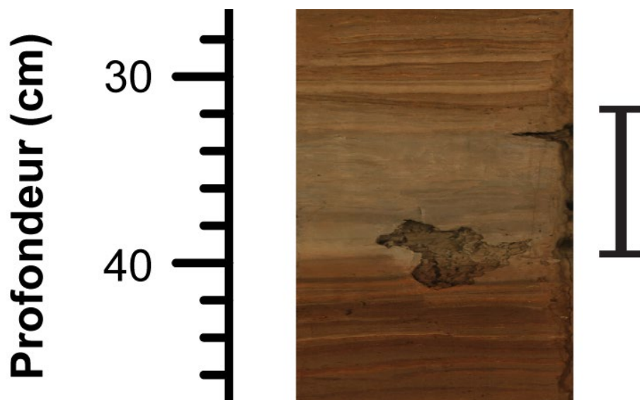
Figure 9.13. Aperçu agrandi des couches de sédiments déposées dans le lac William durant les travaux de vidange du lac Noir (1954–1959 EC). Note : les couches sont délimitées par le marqueur noir (31,75 à 39,5 cm de profondeur). Elles ont été déterminées à partir du modèle chronologique (en considérant les marges d'erreur associées aux dates) et de l'observation de la stratigraphie.
