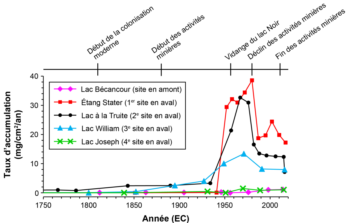
Figure 11.4. Comparaison de l'évolution (1750–2017 EC) des taux d'accumulation d'amiante aux sites de carottage des lacs du bassin de la rivière Bécancour.
