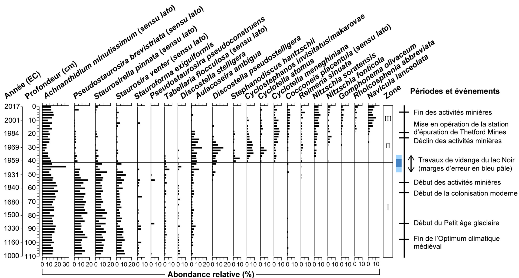
Figure 8.11. Diagramme stratigraphique de l'abondance relative des taxons de diatomées les plus communs ( \geq 4\% dans au moins 1 échantillon) dans la carotte de sédiments du lac à la Truite.
