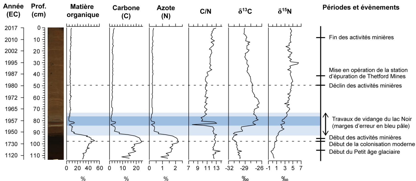
Figure 7.4. Profils de variation des concentrations en matière organique, carbone (C) et azote (N) dans la carotte de sédiments de l'étang Stater. Les rapports du carbone sur l'azote (C/N) et des isotopes stables du carbone 13 sur le carbone 12 ( \delta^{13}\text{C} ) et de l'azote 15 sur l'azote 14 ( \delta^{15}\text{N} ) sont également présentés. Note : les traits pointillés marquent le début de la colonisation moderne de la Haute-Bécancour (~ 1810 EC) et le début du déclin des activités minières d'amiante (1980 EC).
