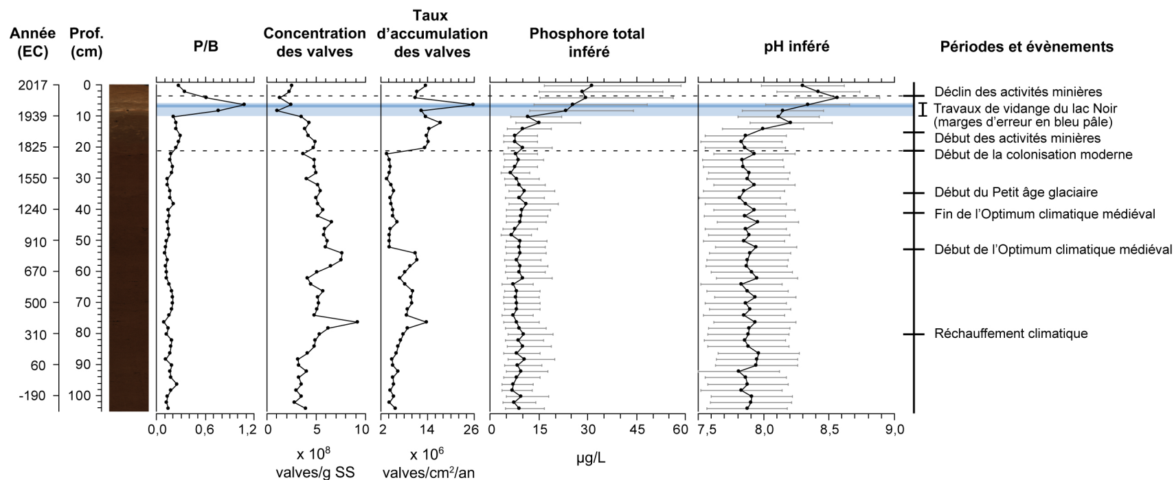
Figure 10.12. Profils de variation du ratio de diatomées planctoniques sur benthiques (P/B) et de la concentration et du taux d'accumulation des valves de diatomées dans la carotte de sédiments du lac Joseph. Les valeurs inférées de phosphore total et de pH basées sur la composition des assemblages sont également présentées. Note : Les traits pointillés marquent le début de la colonisation moderne de la Haute-Bécancour (~ 1810 EC) et le début du déclin des activités minières d'amiante (1980 EC). SS, sédiments secs.
