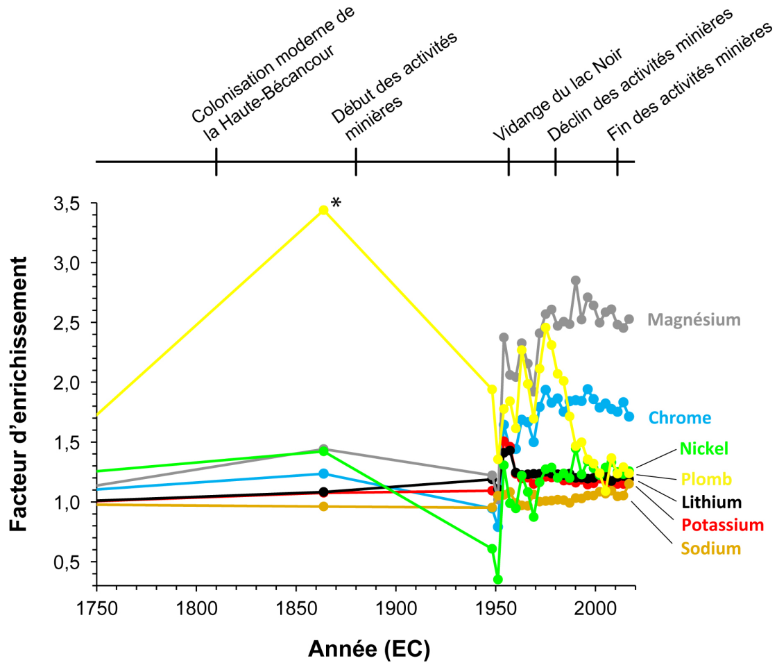
Figure 7.8. Évolution du facteur d'enrichissement de certains métaux sélectionnés dans les sédiments récents de l'étang Stater (1750–2017 EC). Note : les métaux présentés sont ceux ayant les facteurs les plus élevés depuis la colonisation moderne de la Haute-Béancour (~ 1810 EC). * Valeur douteuse.
