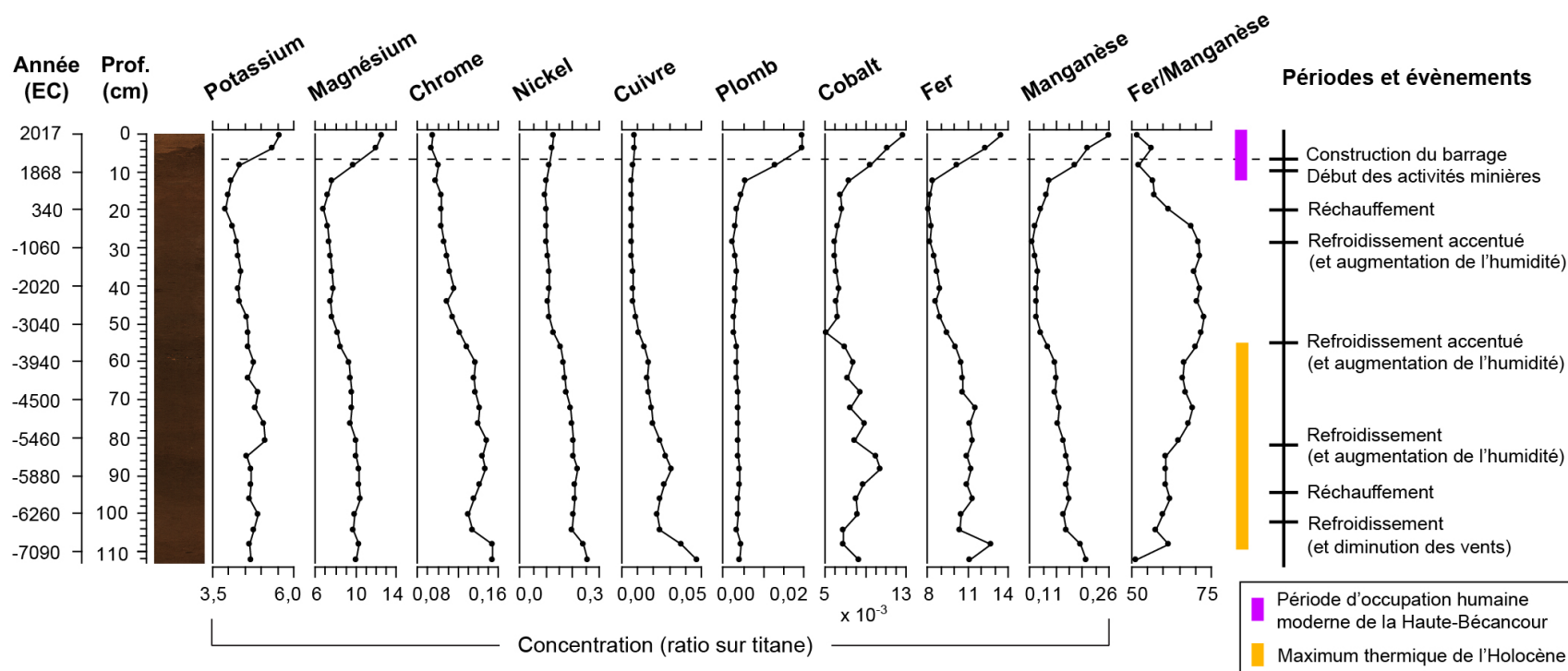
Figure 6.6. Profils de variation de la concentration relative (vis-à-vis le titane ou le manganèse) de certains métaux sélectionnés dans la carotte de sédiments du lac Bécancour. Note : le trait pointillé marque la construction du barrage situé à l'embouchure du plan d'eau (~ 1940 EC).
