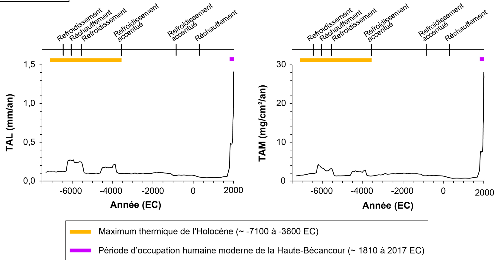
Figure 6.2. Évolution des taux d'accumulation linéaire (TAL; mm/an) et des taux d'accumulation massique (TAM; mg/cm²/an) de sédiments au lac Bécancour.
