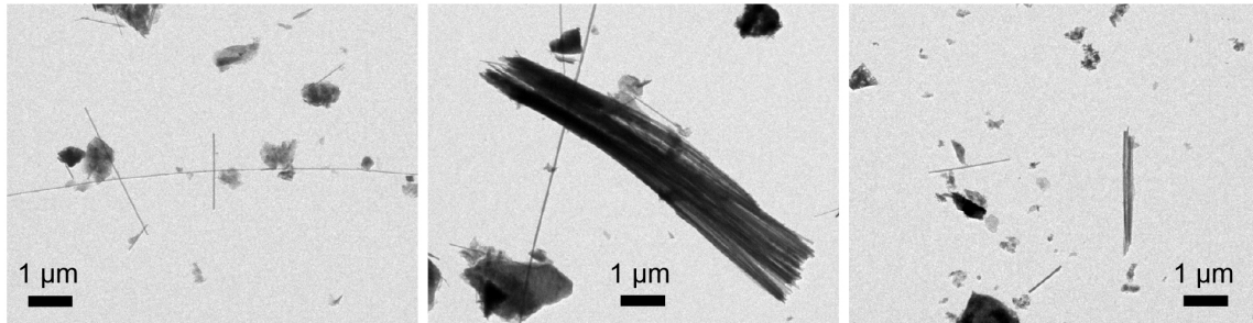
Figure 8.9. Photographies de fibres d’amiante chrysotile présentes aux niveaux 6,5–7,0 cm (gauche), 21,5–22,0 cm (centre) et 94,5–95,0 cm (droite) de la carotte de sédiments du lac à la Truite (grossissement 1100x).
