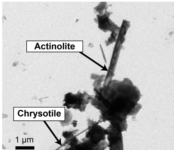
Figure 9.8. Photographie de fibres d'actinolite et de chrysotile présentes au niveau 0,0–1,0 cm de la carotte de sédiments du lac William (grossissement 1100x).
