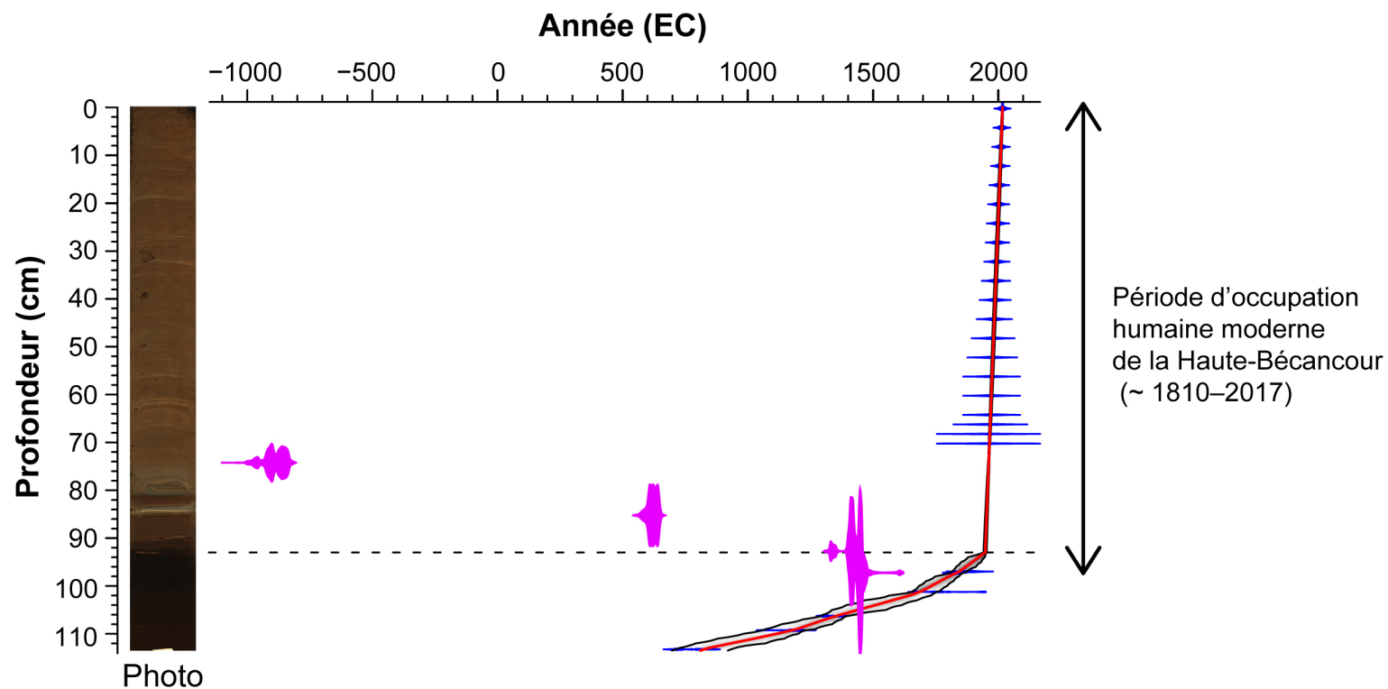
Figure 7.1. Présentation de la carotte de sédiments de l'étang Stater et de son modèle chronologique. Note : la photo illustre l'intérieur de la carotte (plan longitudinal). La ligne rouge représente la courbe d'âge associée aux différents niveaux de profondeurs. Les lignes noires délimitent les intervalles d'erreur (niveau de confiance de 95 %). Les marqueurs bleus désignent les dates qui ont été retenues afin d'établir le modèle, tandis que les marqueurs mauves représentent des dates qui ont été exclues. La ligne pointillée horizontale marque une coupure stratigraphique importante qui a été considérée pour l'élaboration du modèle chronologique.
