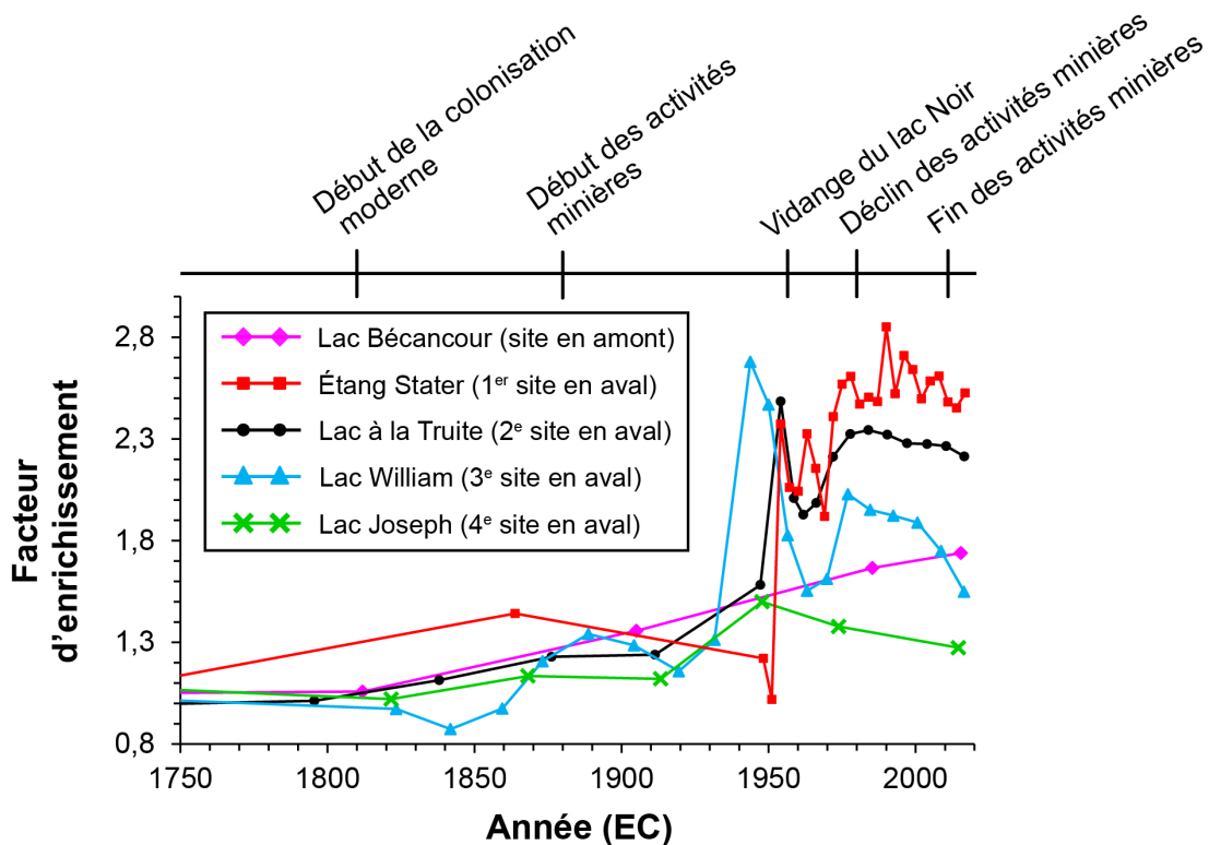
Figure 11.2. Comparaison de l'évolution (1750–2017 EC) du facteur d'enrichissement en magnésium dans les sédiments des lacs du bassin de la rivière Bécancour.
