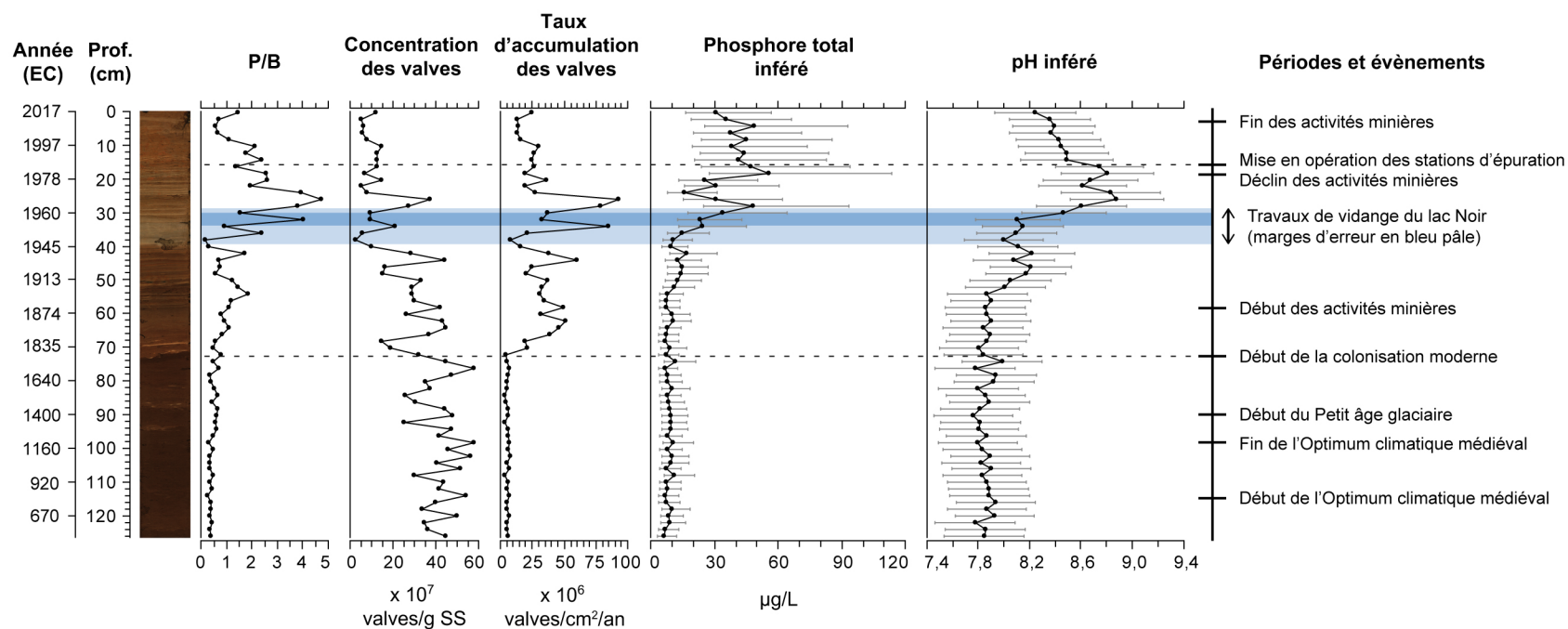
Figure 9.12. Profils de variation du ratio de diatomées planctoniques sur benthiques (P/B) et de la concentration et du taux d’accumulation des valves de diatomées dans la carotte de sédiments du lac William. Les valeurs inférées de phosphore total et de pH basées sur la composition des assemblages sont également présentées. Note : SS, sédiments secs. Les traits pointillés marquent le début de la colonisation moderne de la Haute-Bécancour (~ 1810 EC) et la mise en opération des stations d’épuration de Saint-Ferdinand et Thetford Mines (1985–1986 EC).
