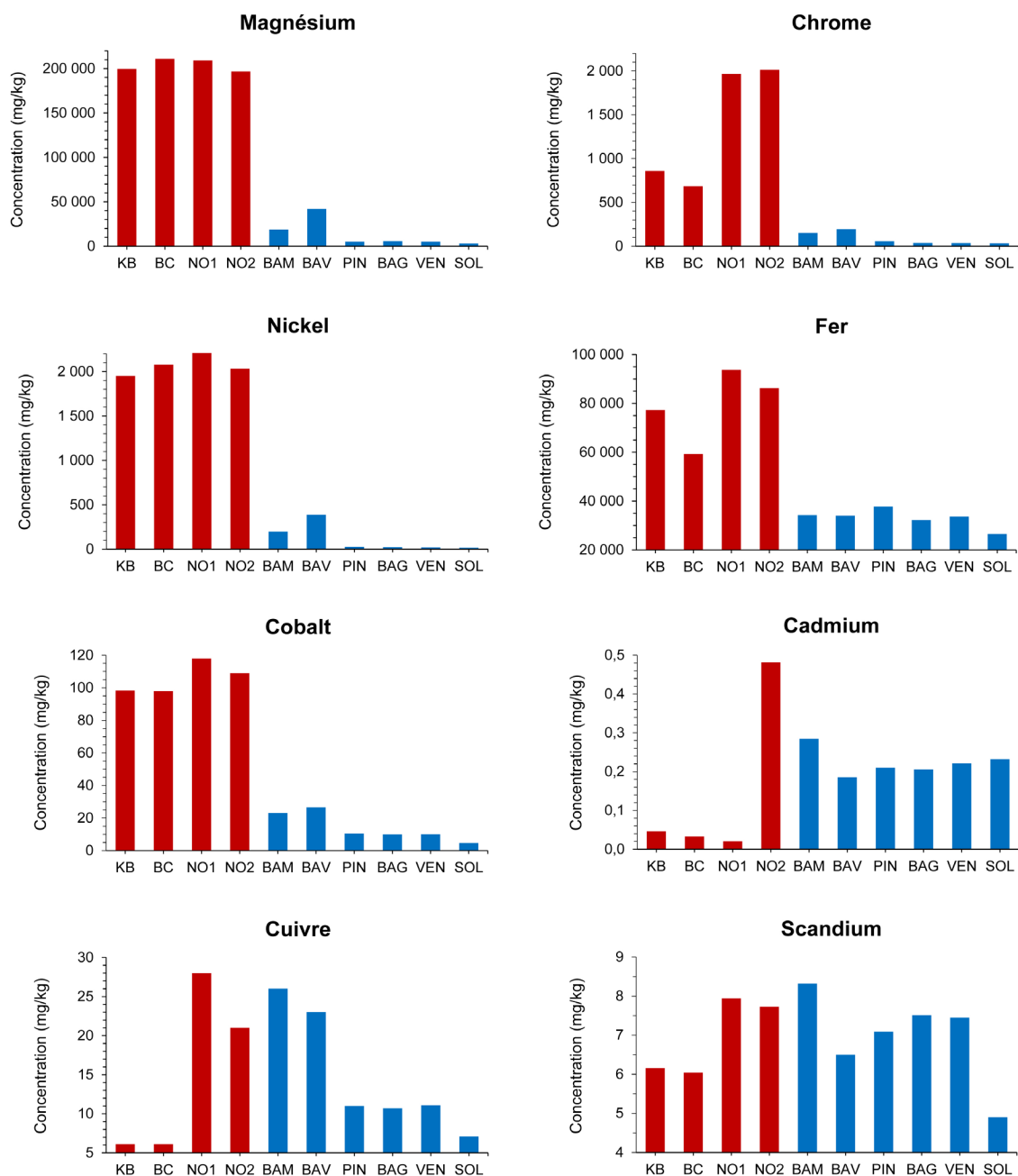
Figure 5.1. Teneurs en éléments chimiques des échantillons de sources sédimentaires de la Haute-Bécancour. Note : les bandes rouges désignent les échantillons de résidus miniers amiantés, tandis que les bandes bleues désignent les autres types d'échantillons (sédiments de rivière et sol). BAG, rivière Bagot; BAM, rivière Bécancour – amont des haldes; BAV, rivière Bécancour – aval des haldes; BC, mine British Canadian 1; KB, mine King-Beaver; NO1, échantillon #1 de la mine Normandie; NO2, échantillon #2 de la mine Normandie (prélevé sur la berge de la rivière Bécancour); PIN, rivière au Pin; SOL, sol en bordure du lac à la Truite; VEN, ruisseau Venlo.
