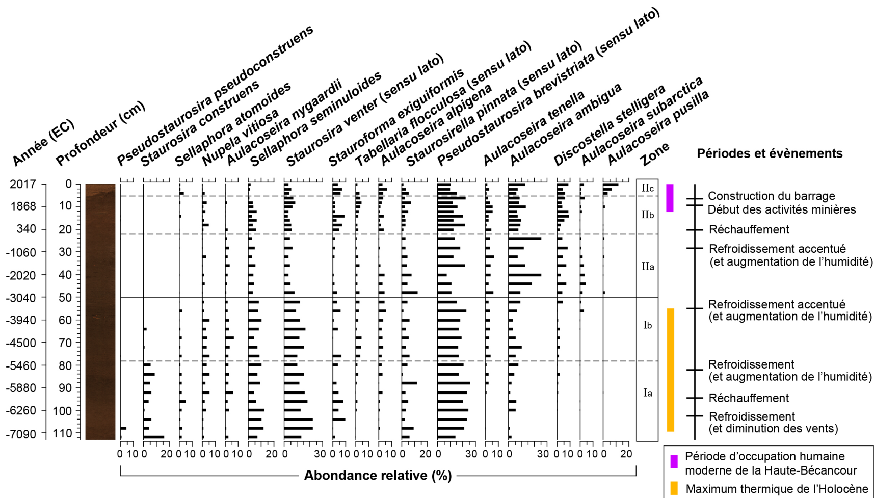
Figure 6.11. Diagramme stratigraphique de l'abondance relative des taxons de diatomées les plus communs ( \geq 4\% dans au moins 1 échantillon) dans la carotte de sédiments du lac Bécancour.
