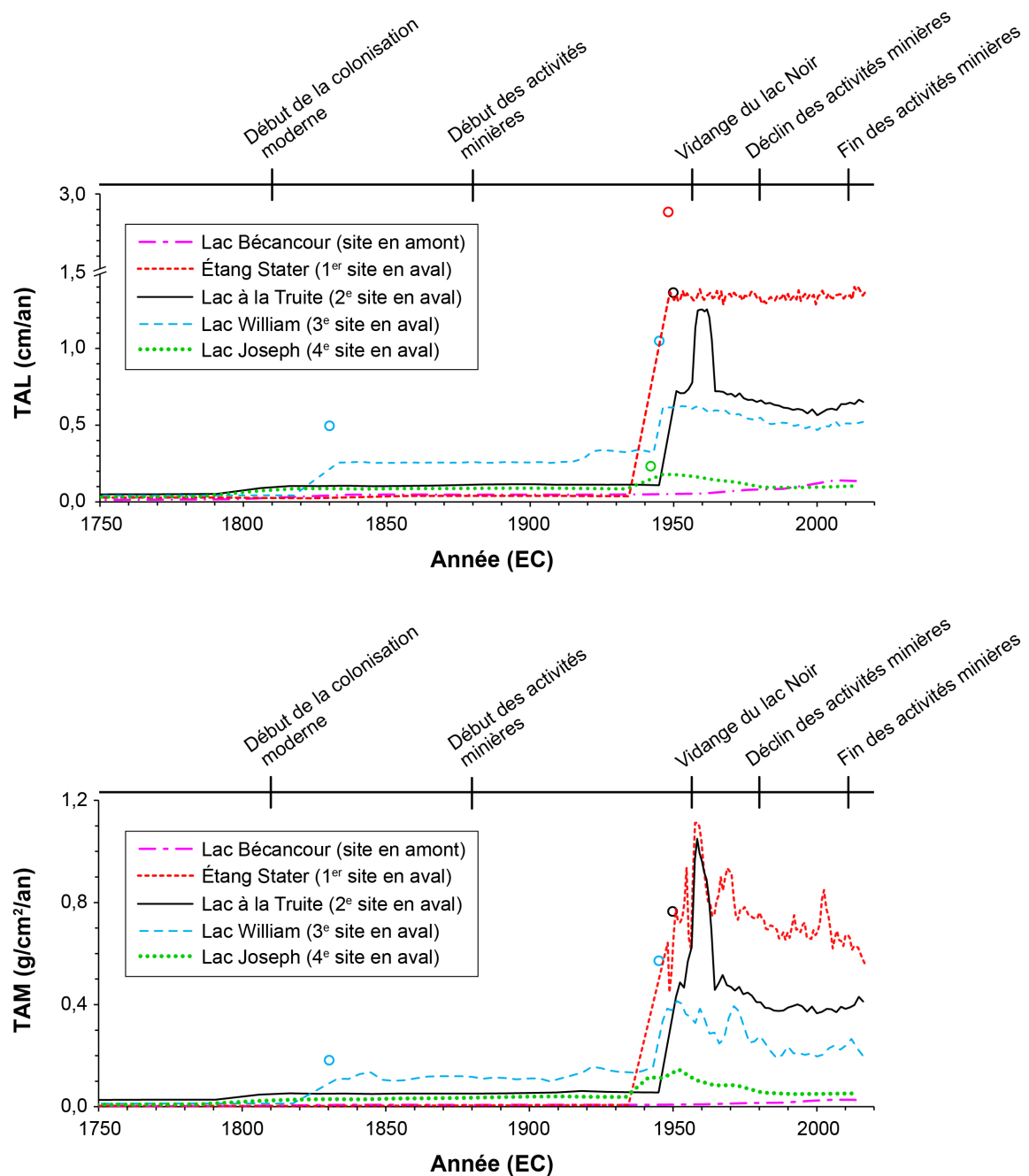
Figure 11.1. Comparaison de l'évolution (1750–2017 EC) des taux d'accumulation linéaire (TAL; graphique supérieur) et des taux d'accumulation massique (TAM; graphique inférieur) de sédiments aux sites de carottage des lacs du bassin de la rivière Bécancour. Note : les cercles vides représentent des valeurs aberrantes qui ont été exclues.
