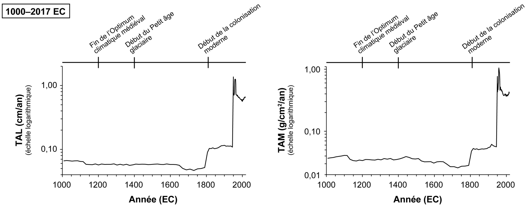
Figure 8.2. Évolution des taux d'accumulation linéaire (TAL; cm/an) et des taux d'accumulation massique (TAM; g/cm 2 /an) de sédiments au lac à la Truite.
