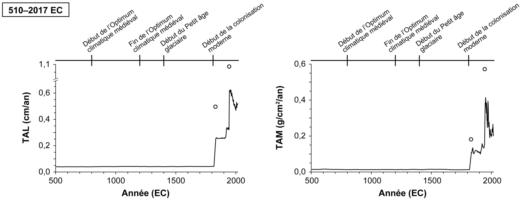
Figure 9.2. Évolution des taux d'accumulation linéaire (TAL; cm/an) et des taux d'accumulation massique (TAM; g/cm 2 /an) de sédiments au lac William. Note : les cercles vides désignent des valeurs aberrantes qui ont été exclues.
