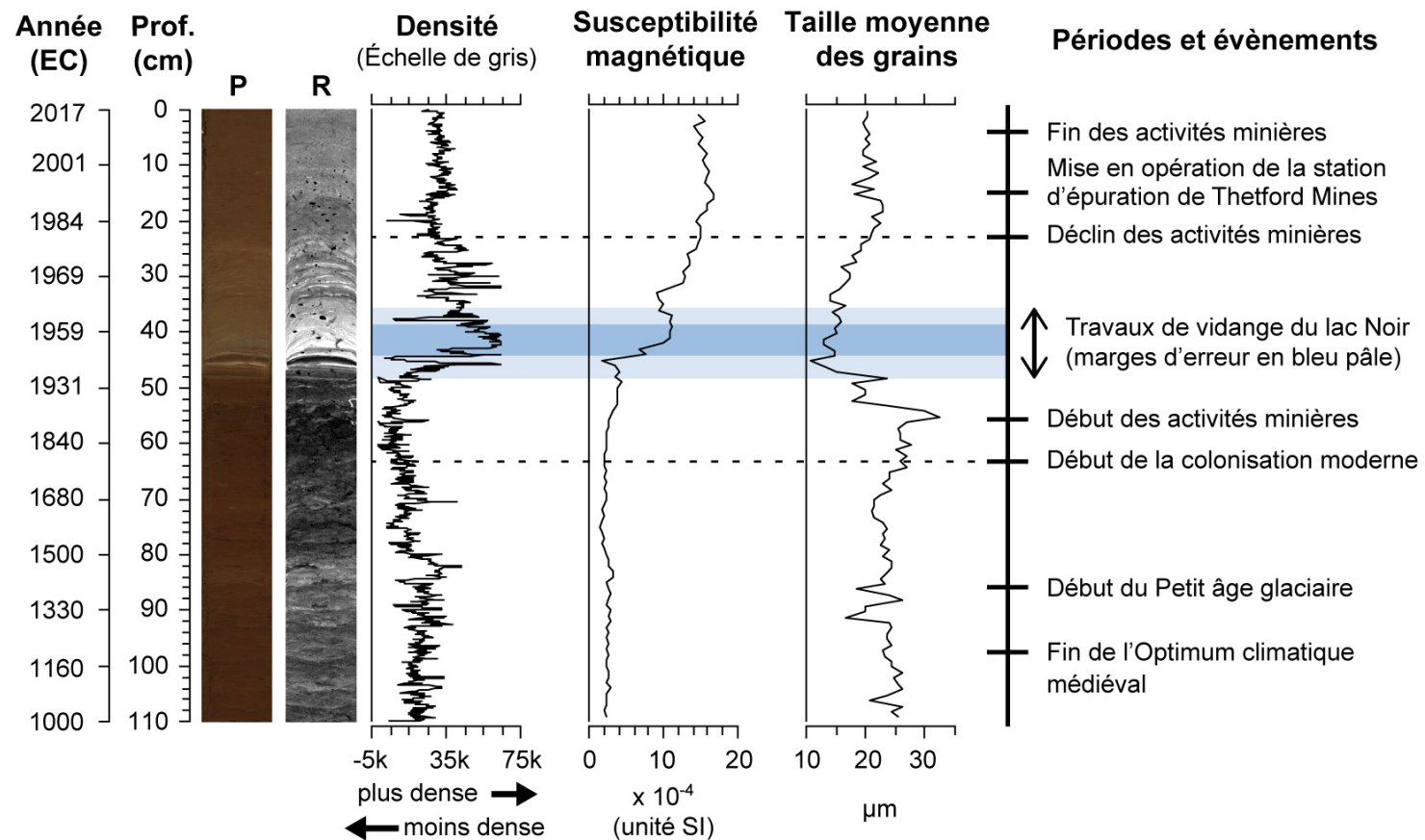
Figure 8.3. Profils de variation de la densité, de la susceptibilité magnétique et de la taille moyenne des grains dans la carotte de sédiments du lac à la Truite. Note : les traits pointillés marquent le début de la colonisation moderne de la Haute-Béancour (~ 1810 EC) et le début du déclin des activités minières d'amiante (1980 EC). P, photographie; R, radiographie.
