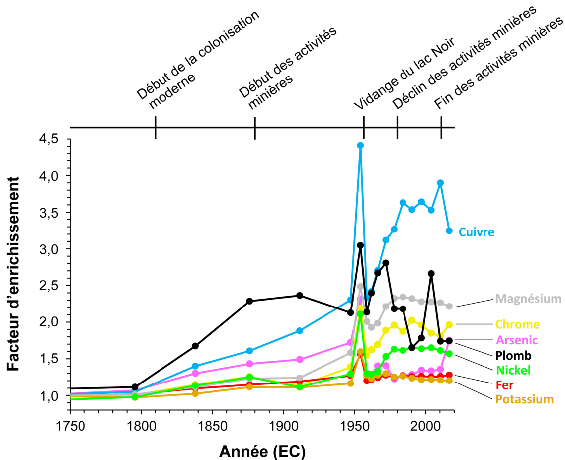
Figure 8.7. Évolution du facteur d'enrichissement de certains métaux sélectionnés dans les sédiments récents du lac à la Truite (1750–2017 EC). Note : les métaux présentés sont ceux ayant les facteurs les plus élevés depuis la colonisation moderne de la Haute-Bécancour (~ 1810 EC).
