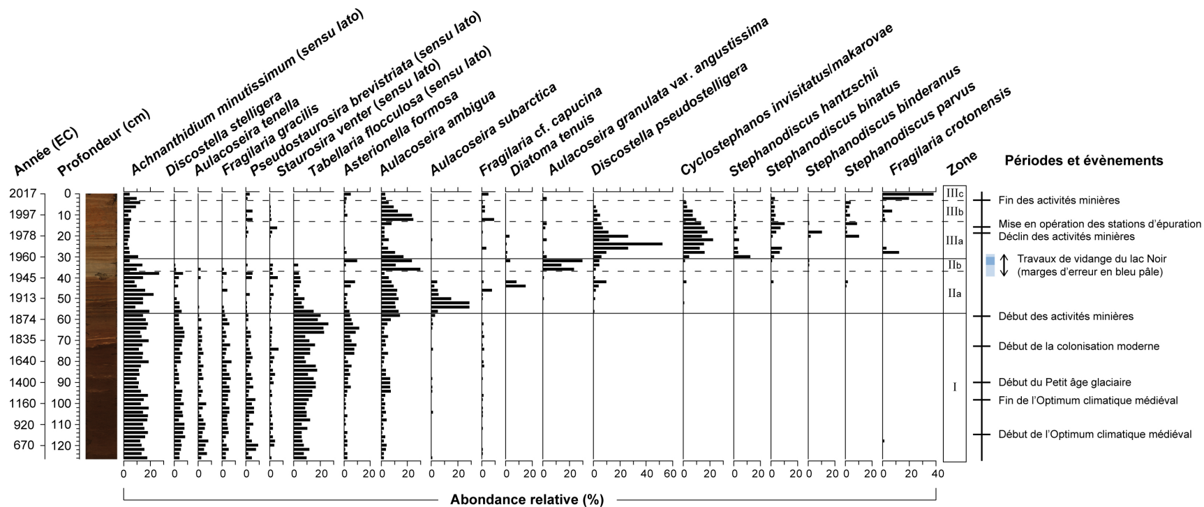
Figure 9.11. Diagramme stratigraphique de l'abondance relative des taxons de diatomées les plus communs ( \geq 7\% dans au moins 1 échantillon) dans la carotte de sédiments du lac William.
