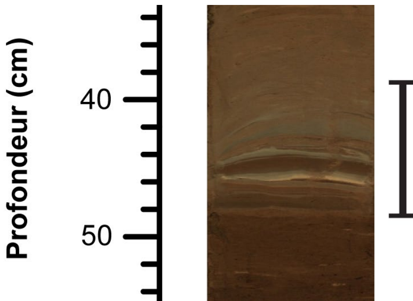
Figure 8.13. Aperçu agrandi des couches de sédiments déposées dans le lac à la Truite durant les travaux de vidange du lac Noir (1954–1959 EC). Note : les couches sont délimitées par le marqueur noir (38,75 à 48,5 cm de profondeur). Elles ont été déterminées à partir du modèle chronologique (en considérant les marges d'erreur associées aux dates) et de l'observation de la stratigraphie.
