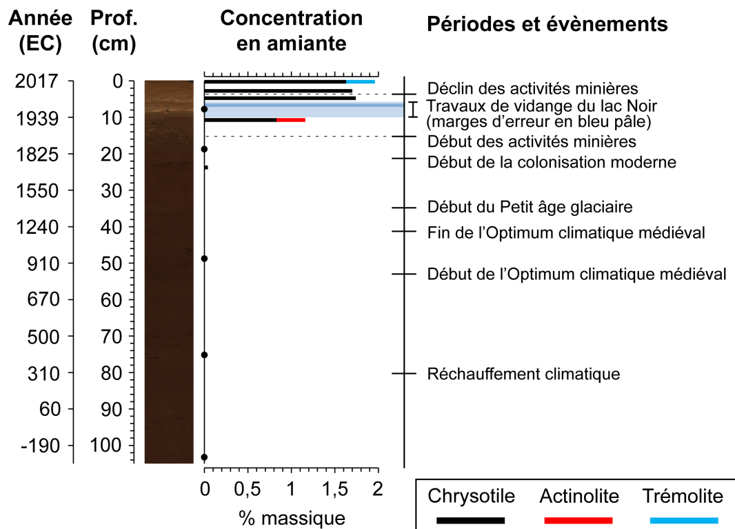
Figure 10.9. Concentration en fibres d'amiante à différents niveaux de profondeur de la carotte de sédiments du lac Joseph. Note : les traits pointillés marquent le début des activités minières d'amiante dans la Haute-Bécancour (~ 1880 EC) et le début du déclin de l'industrie minière régionale (1980 EC).
