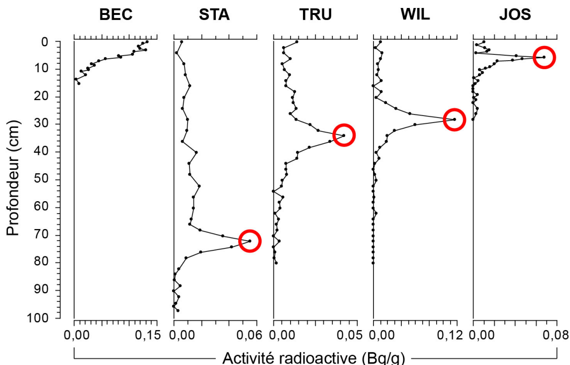
Figure 4.6. Profils de variation de l'activité radioactive du césium 137 ( ^{137}\text{Cs} ) dans les carottes de sédiments du lac Bécancour (BEC), de l'étang Stater (STA), du lac à la Truite (TRU), du lac William (WIL) et du lac Joseph (JOS). Note : les cercles rouges désignent des pics importants qui ont été associés au maximum des tests d'armement nucléaire de 1963.
