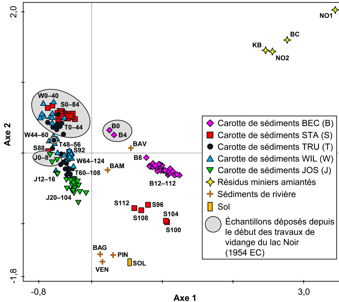
Figure 11.3. Analyse en composantes principales permettant de comparer la composition géochimique des différentes couches des carottes de sédiments et des échantillons de sources de matériel sédimentaire présentes dans la Haute-Bécancour. Note : la position des marqueurs est déterminée en fonction de leur composition en métaux (aluminium, baryum, calcium, cadmium, cobalt, chrome, cuivre, potassium, lithium, magnésium, nickel, scandium, sodium, strontium, titane et zinc). Certains éléments chimiques n'ont pas été considérés puisque leur abondance dans les sédiments est particulièrement dépendante d'apports atmosphériques et de conditions d'oxygénation (arsenic, fer, manganèse, plomb, phosphore et soufre). Sur le graphique, les chiffres associés aux échantillons des carottes de sédiments représentent leur profondeur arrondie en centimètres (p. ex., B12-112 = profondeurs allant de 12 à 112 cm dans la carotte de sédiments du lac Bécancour). BAG, rivière Bagot; BAM, rivière Bécancour – en amont des halles minières; BAV, rivière Bécancour – en aval des halles minières; KB, mine King-Beaver; BC, mine British Canadian 1; NO1, mine Normandie – échantillon #1 (prélevé au bas des halles); NO2, mine Normandie – échantillon #2 (prélevé sur le bord de la rivière Bécancour); PIN, rivière au Pin; SOL, sol adjacent au lac à la Truite; VEN, ruisseau Venlo.
