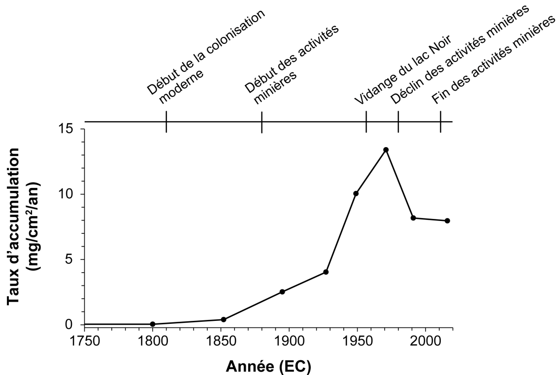
Figure 9.10. Évolution du taux d'accumulation de fibres d'amiante dans les sédiments récents du lac William (1750–2017 EC).
