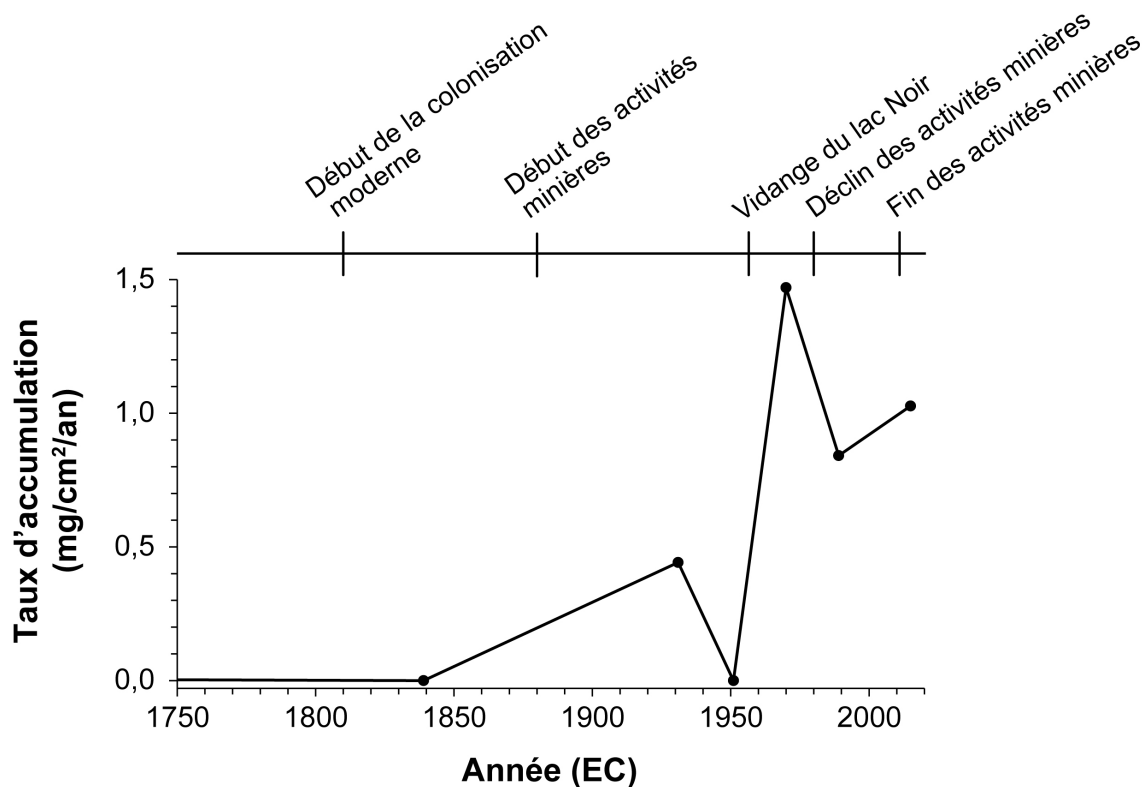
Figure 10.10. Évolution du taux d'accumulation de fibres d'amiante dans les sédiments récents du lac Joseph (1750–2017 EC).
