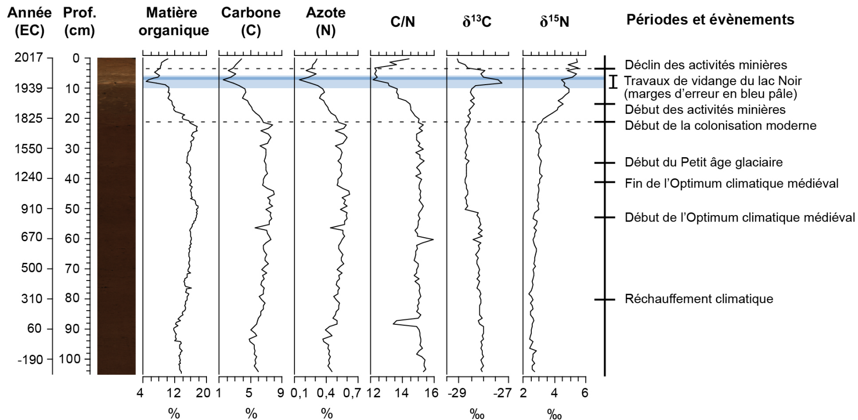
Figure 10.4. Profils de variation des concentrations en matière organique, carbone (C) et azote (N) dans la carotte de sédiments du lac Joseph. Les rapports du carbone sur l'azote (C/N) et des isotopes stables du carbone 13 sur le carbone 12 ( \delta^{13}\text{C} ) et de l'azote 15 sur l'azote 14 ( \delta^{15}\text{N} ) sont également présentés. Note : les traits pointillés marquent le début de la colonisation moderne de la Haute-Bécancour (~ 1810 EC) et le début du déclin des activités minières d'amiante (1980 EC).
