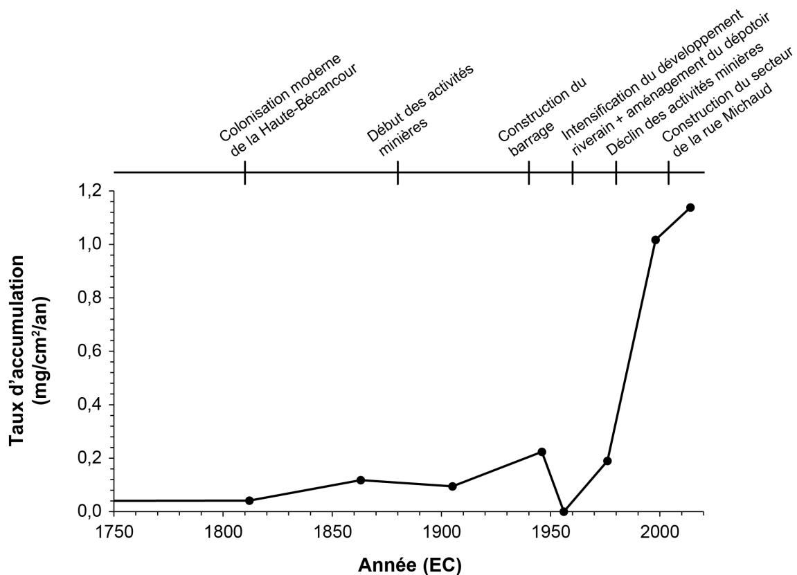
Figure 6.10. Évolution du taux d'accumulation de fibres d'amiante dans les sédiments récents du lac Bécancour (1750–2017 EC).
