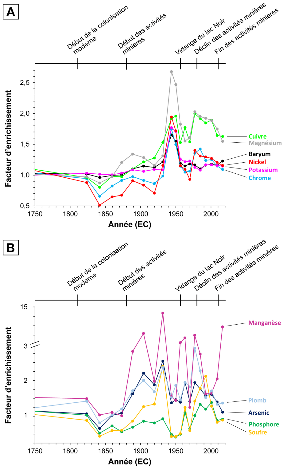
Figure 9.7. Évolution du facteur d'enrichissement de certains métaux sélectionnés dans les sédiments récents du lac William (1750–2017 EC). Note : les métaux présentés sont ceux ayant les facteurs les plus élevés depuis la colonisation moderne de la Haute-Béancour (~ 1810 EC). Ils sont groupés selon leur patron de variation : A) cuivre, magnésium, baryum, nickel, potassium et chrome; B) manganèse, plomb, arsenic, phosphore et soufre.
