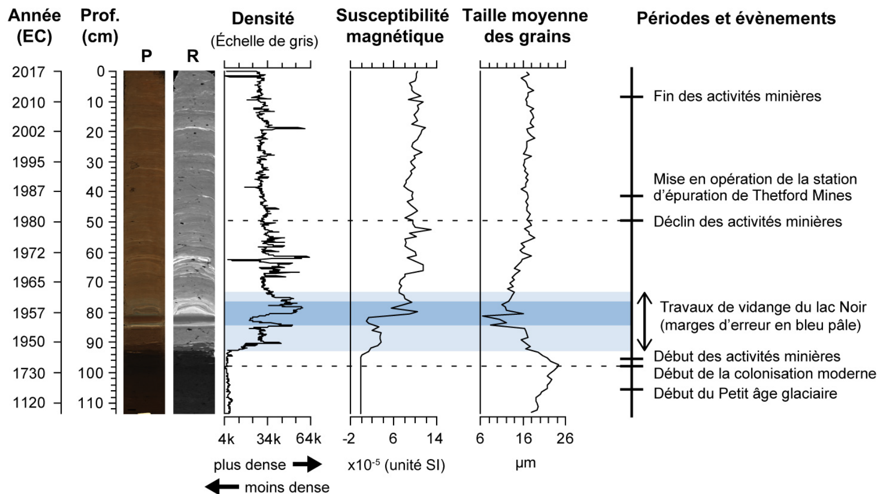
Figure 7.3. Profils de variation de la densité, de la susceptibilité magnétique et de la taille moyenne des grains dans la carotte de sédiments de l'étang Stater. Note : les traits pointillés marquent le début de la colonisation moderne de la Haute-Bécancour (~ 1810 EC) et le début du déclin des activités minières d'amiante (1980 EC).
