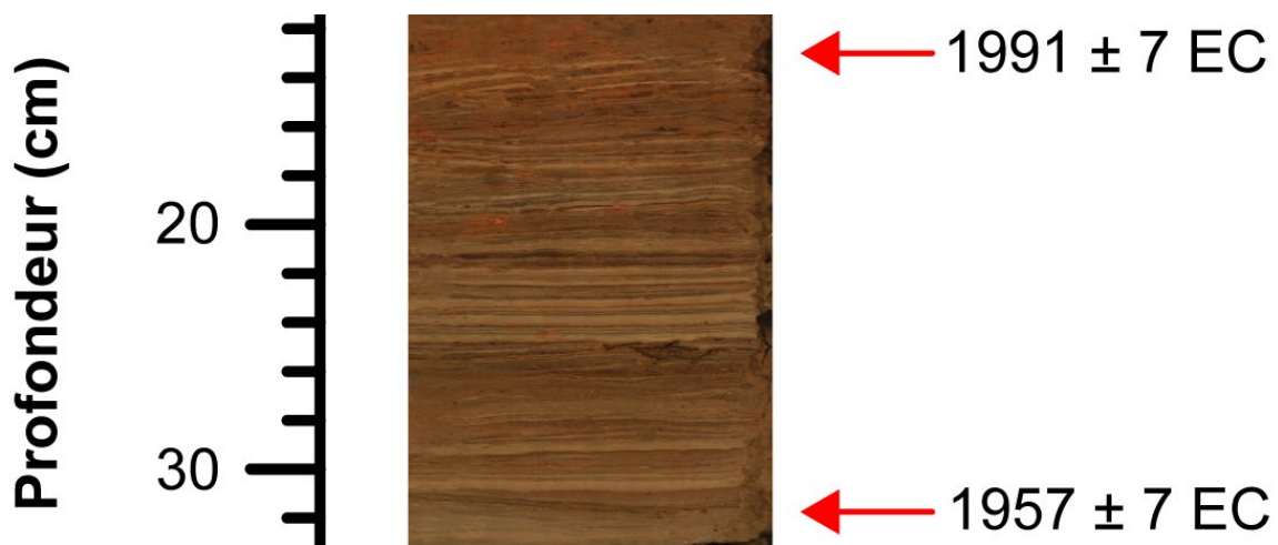
Figure 9.14. Aperçu agrandi des laminations fines (minces couches de sédiments) préservées dans la stratigraphie des années 1957 \pm 7 à 1991 \pm 7 EC (31,75 à 13 cm) du lac William.
