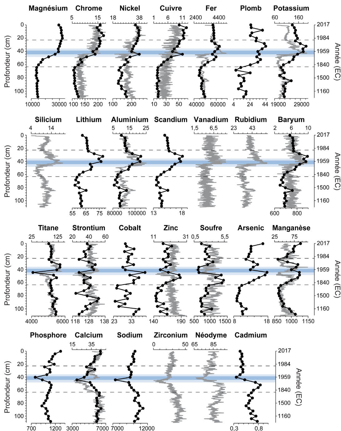
Figure 8.5. Profils de variation de la concentration absolue en métaux et autres éléments chimiques dans la carotte de sédiments du lac à la Truite. Note : les courbes et points noirs (axes horizontaux inférieurs) représentent les données de concentrations (en mg/kg) établies par spectrométrie, tandis que les courbes grises (axes horizontaux supérieurs) correspondent aux données de concentrations relatives obtenues par microfluorescence X. Les zones colorées délimitent la période de travaux de vidange du lac Noir (1954–1959 EC; marges d’erreur en bleu pâle), tandis que les traits pointillés inférieur et supérieur marquent respectivement le début de la colonisation moderne de la Haute-Bécancour (~ 1810 EC) et le début du déclin des activités minières d’amiante (1980 EC).
