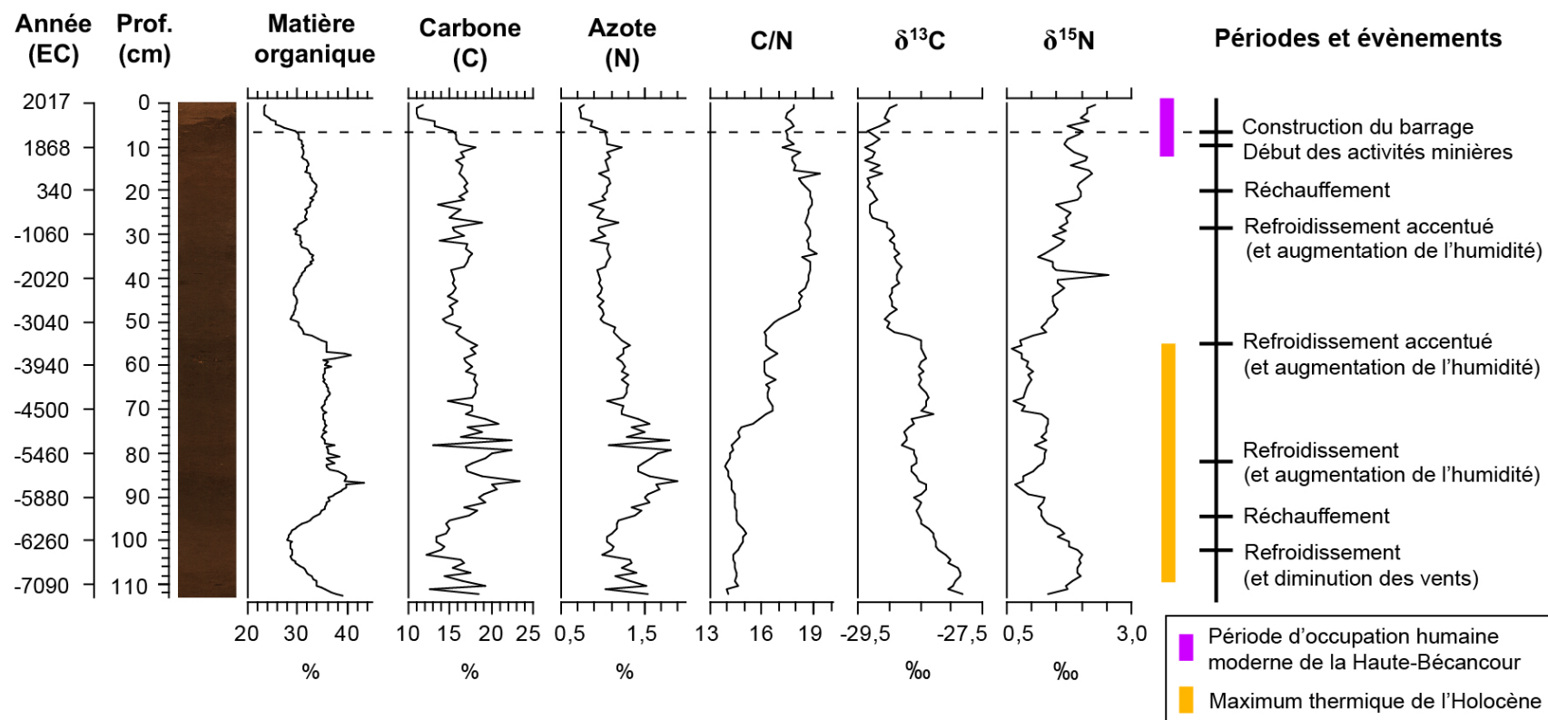
Figure 6.4. Profils de variation des concentrations en matière organique, carbone (C) et azote (N) dans la carotte de sédiments du lac Bécancour. Les rapports du carbone sur l'azote (C/N) et des isotopes stables du carbone 13 sur le carbone 12 ( \delta^{13}\text{C} ) et de l'azote 15 sur l'azote 14 ( \delta^{15}\text{N} ) sont également présentés. Note : le trait pointillé marque la construction du barrage situé à l'embouchure du plan d'eau (~1940 EC).
