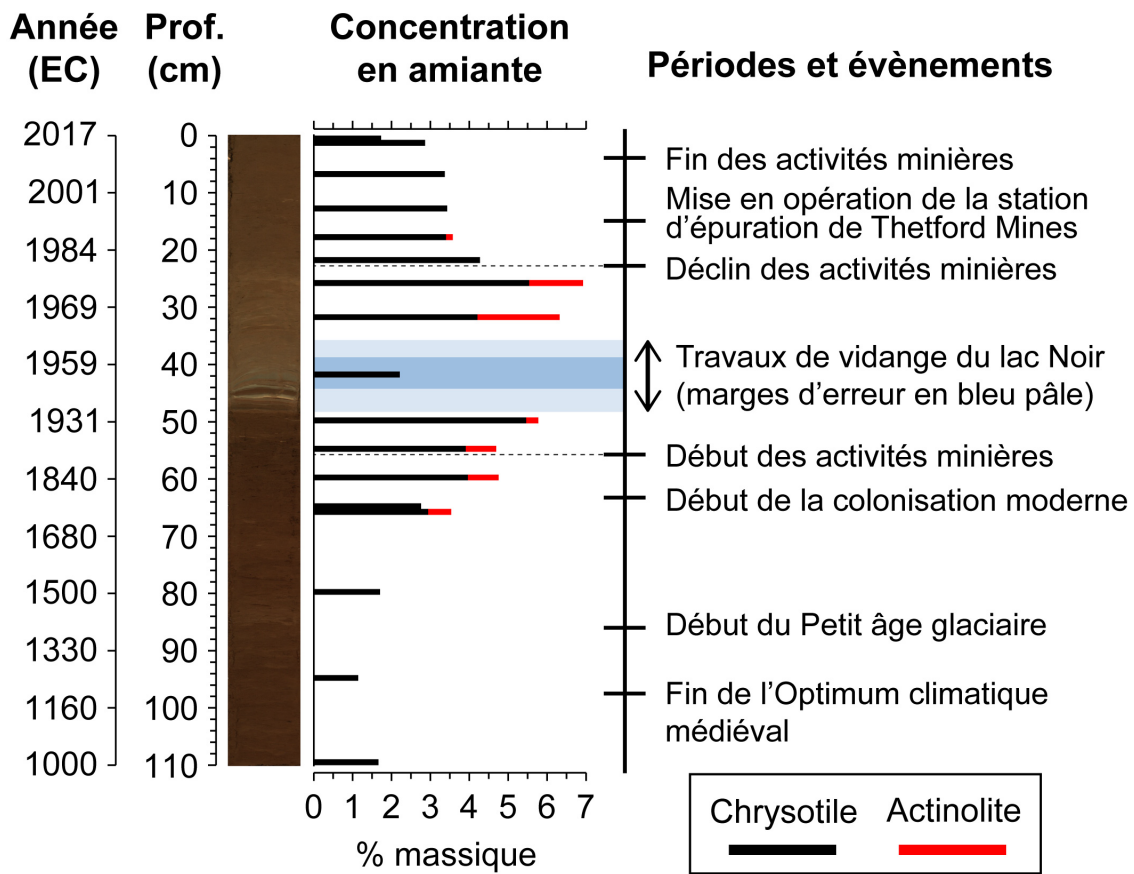
Figure 8.8. Concentration en fibres d’amiante à différents niveaux de profondeur de la carotte de sédiments du lac à la Truite. Note : les traits pointillés marquent le début des activités minières d’amiante dans la Haute-Bécancour (~ 1880 EC) et le début du déclin de l’industrie minière régionale (1980 EC).
