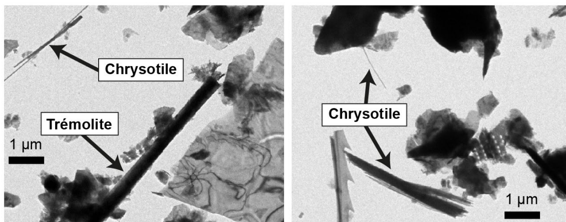
Figure 10.8. Photographies de fibres de trémolite et de chrysotile présentes au niveau 0,0–0,5 cm de la carotte de sédiments du lac Joseph (grossissement 1100x).
