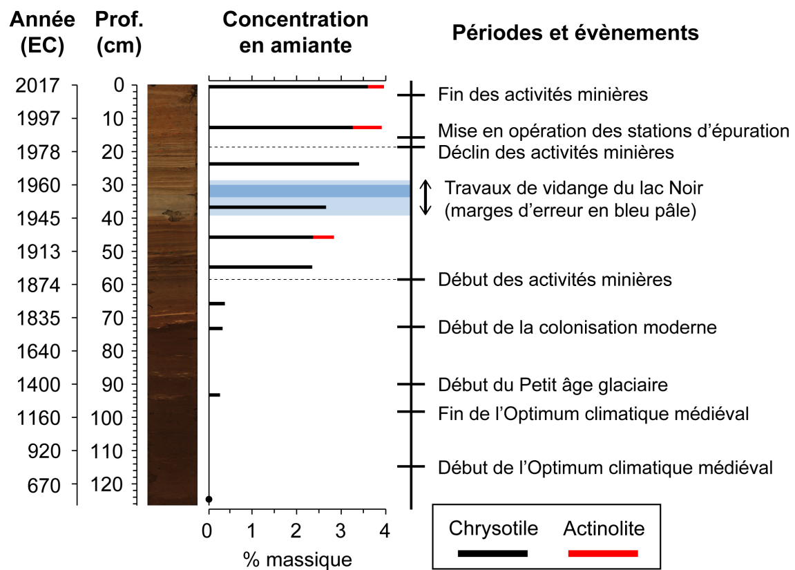
Figure 9.9. Concentration en fibres d'amiante à différents niveaux de profondeur de la carotte de sédiments du lac William. Note : les traits pointillés marquent le début des activités minières d'amiante dans la Haute-Bécancour (~ 1880 EC) et le début du déclin de l'industrie minière régionale (1980 EC).
