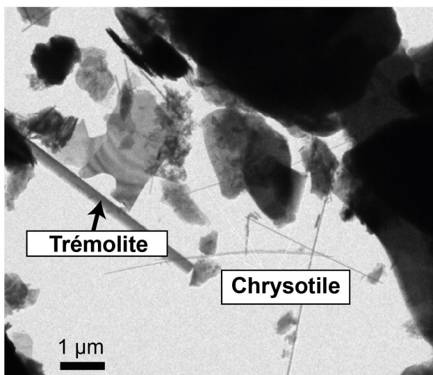
Figure 7.7. Photographie de fibres de trémolite et de chrysotile présentes au niveau 0,0–1,0 cm de la carotte de sédiments de l'étang Stater (grossissement 1100x).
