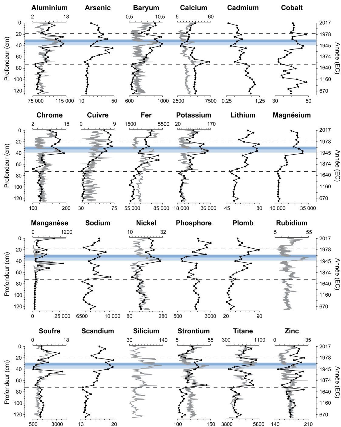
Figure 9.5. Profils de variation de la concentration absolue en métaux et autres éléments chimiques dans la carotte de sédiments du lac William. Note : les courbes et points noirs (axes horizontaux inférieurs) représentent les données de concentrations (en mg/kg) établies par spectrométrie, tandis que les courbes grises (axes horizontaux supérieurs) correspondent aux données de concentrations relatives obtenues par microfluorescence X. Les zones colorées délimitent la période de travaux de vidange du lac Noir (1954–1959 EC; marges d'erreur en bleu pâle), tandis que les traits pointillés inférieur et supérieur marquent respectivement le début de la colonisation moderne de la Haute-Bécancour (~ 1810 EC) et le début du déclin des activités minières d'amiante (1980 EC).
