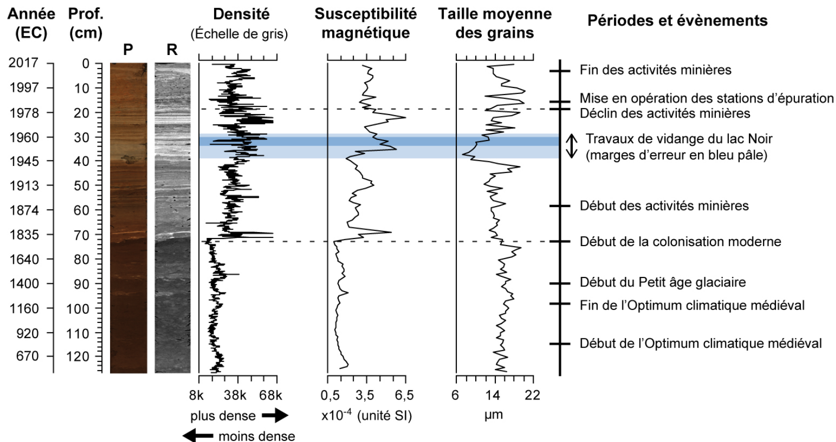
Figure 9.3. Profils de variation de la densité, de la susceptibilité magnétique et de la taille moyenne des grains dans la carotte de sédiments du lac William. Note : les traits pointillés marquent le début de la colonisation moderne de la Haute-Bécancour (~ 1810 EC) et le début du déclin des activités minières d'amiante (1980 EC). P, photographie; R, radiographie.
