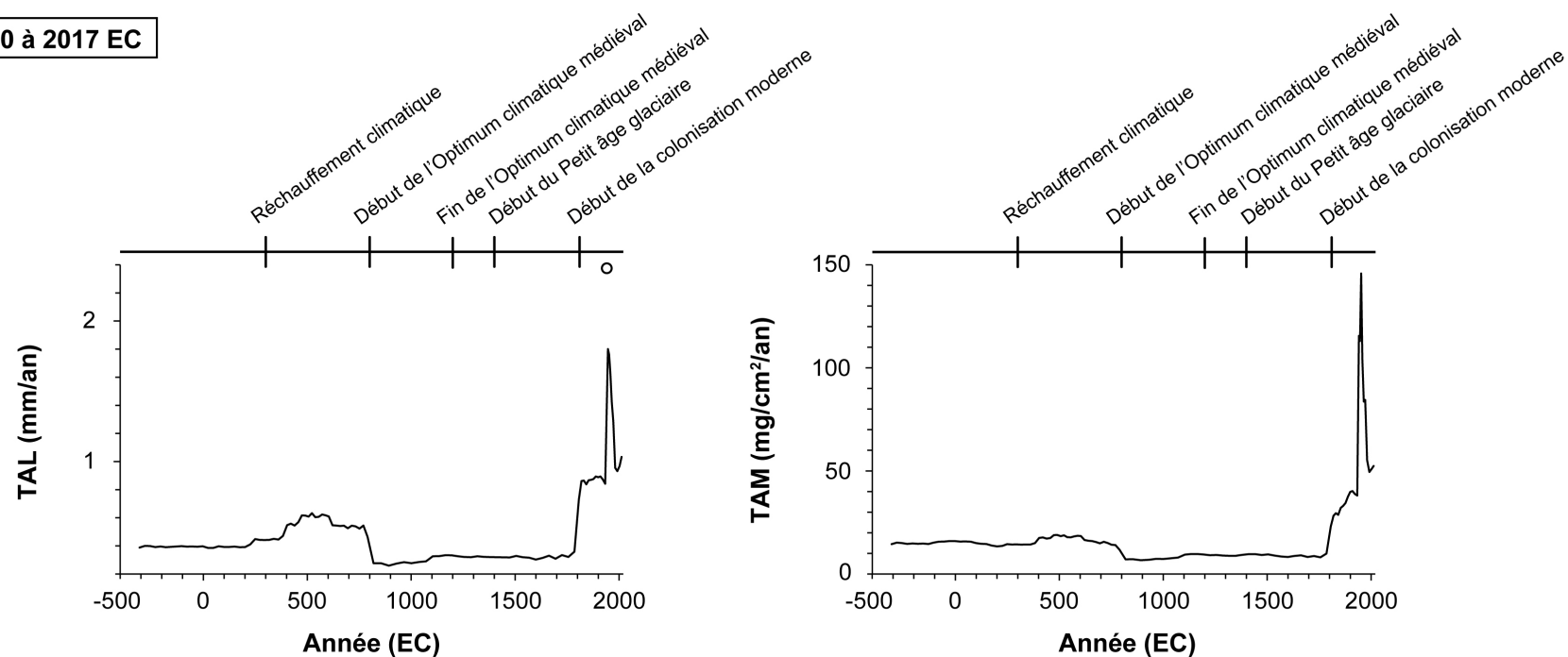
Figure 10.2. Évolution des taux d'accumulation linéaire (TAL; mm/an) et des taux d'accumulation massique (TAM; mg/cm 2 /an) de sédiments au lac Joseph. Note : les cercles vides désignent des valeurs aberrantes qui ont été exclues.
