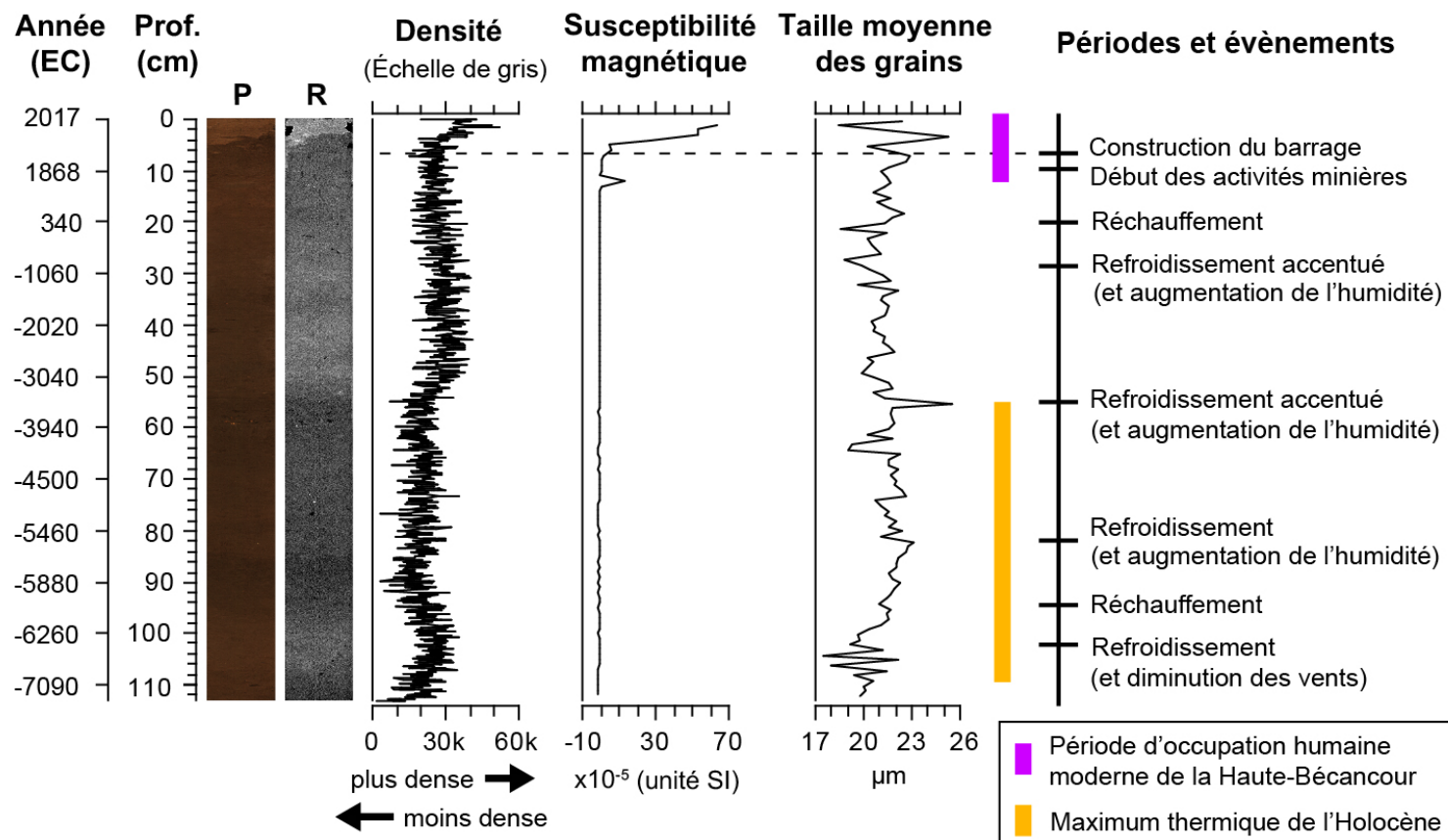
Figure 6.3. Profils de variation de la densité, de la susceptibilité magnétique et de la taille moyenne des grains dans la carotte de sédiments du lac Bécancour.
