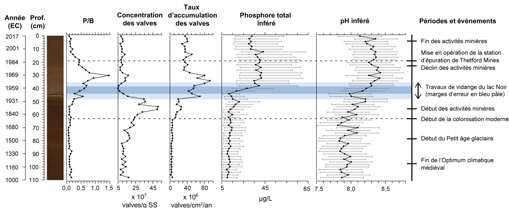
Figure 8.12. Profils de variation du ratio de diatomées planctoniques sur benthiques (P/B) et de la concentration et du taux d'accumulation des valves de diatomées dans la carotte de sédiments du lac à la Truite. Les valeurs inférées de phosphore total et de pH basées sur la composition des assemblages sont également présentées. Note : Les traits pointillés marquent le début de la colonisation moderne de la Haute-Bécancour (~ 1810 EC) et le début du déclin des activités minières d'amiante (1980 EC). SS, sédiments secs.
