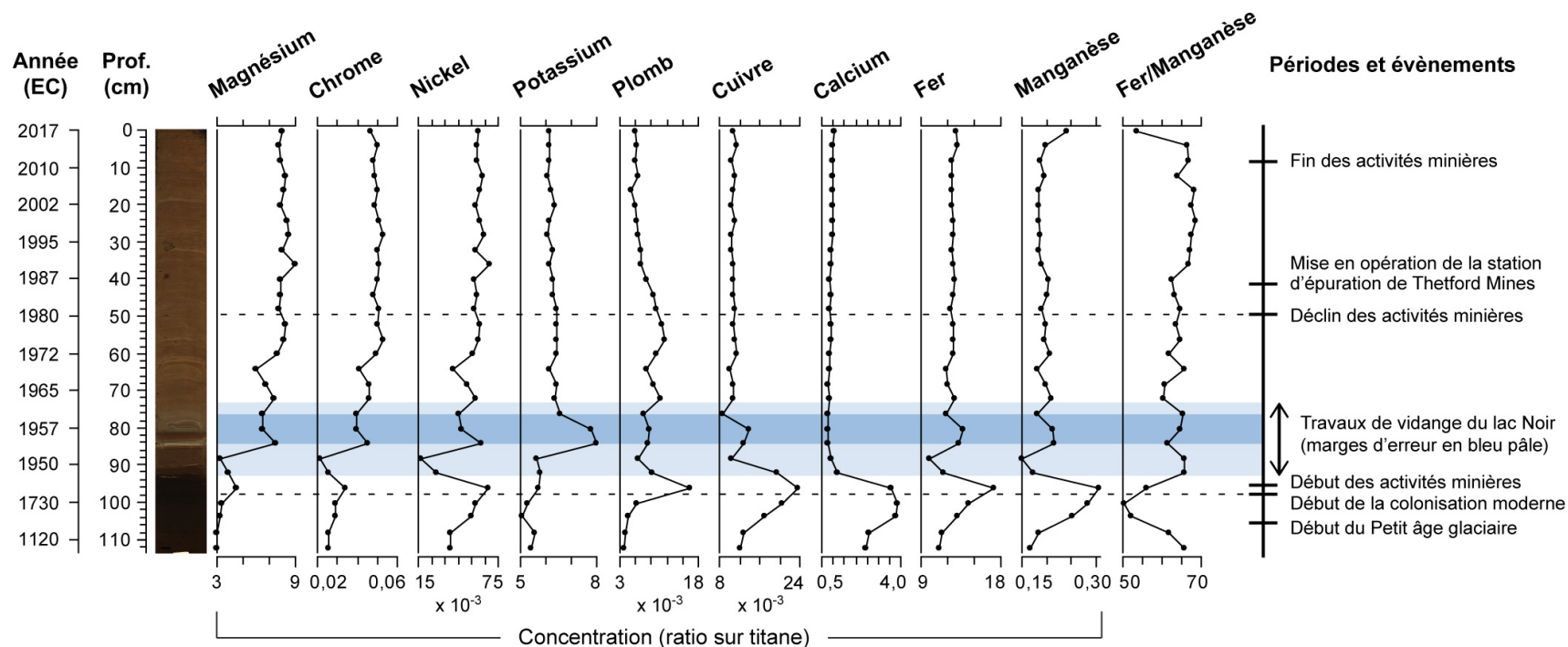
Figure 7.6. Profils de variation de la concentration relative (vis-à-vis le titane ou le manganèse) de certains métaux dans la carotte de sédiments de l'étang Stater. Note : les traits pointillés marquent le début de la colonisation moderne de la Haute-Bécancour (~ 1810 EC) et le début du déclin des activités minières d'amiante (1980 EC).
