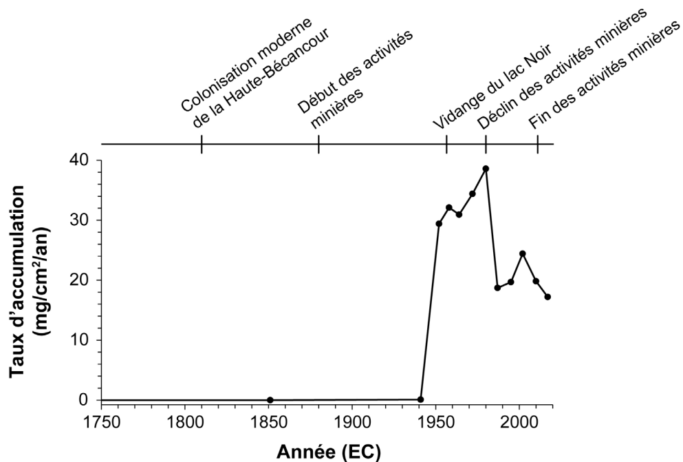
Figure 7.10. Évolution du taux d'accumulation de fibres d'amiante dans les sédiments récents de l'étang Stater (1750–2017 EC).
