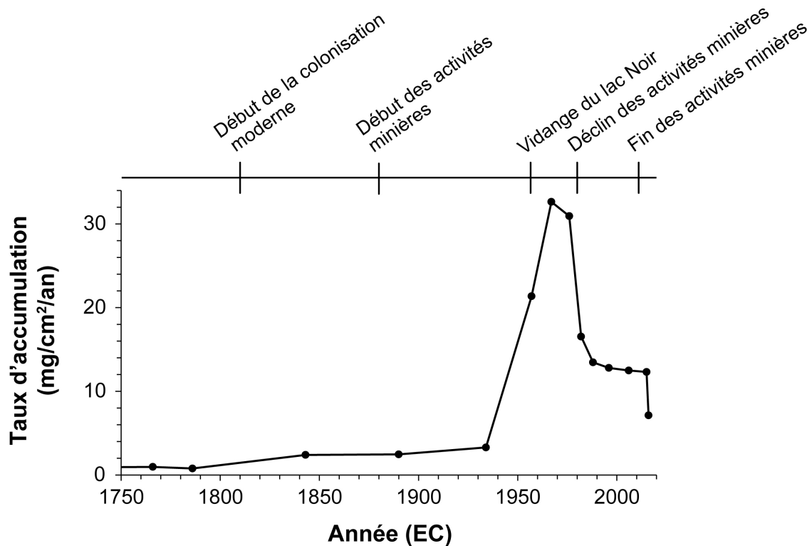
Figure 8.10. Évolution du taux d'accumulation de fibres d'amiante dans les sédiments récents du lac à la Truite (1750–2017 EC).
