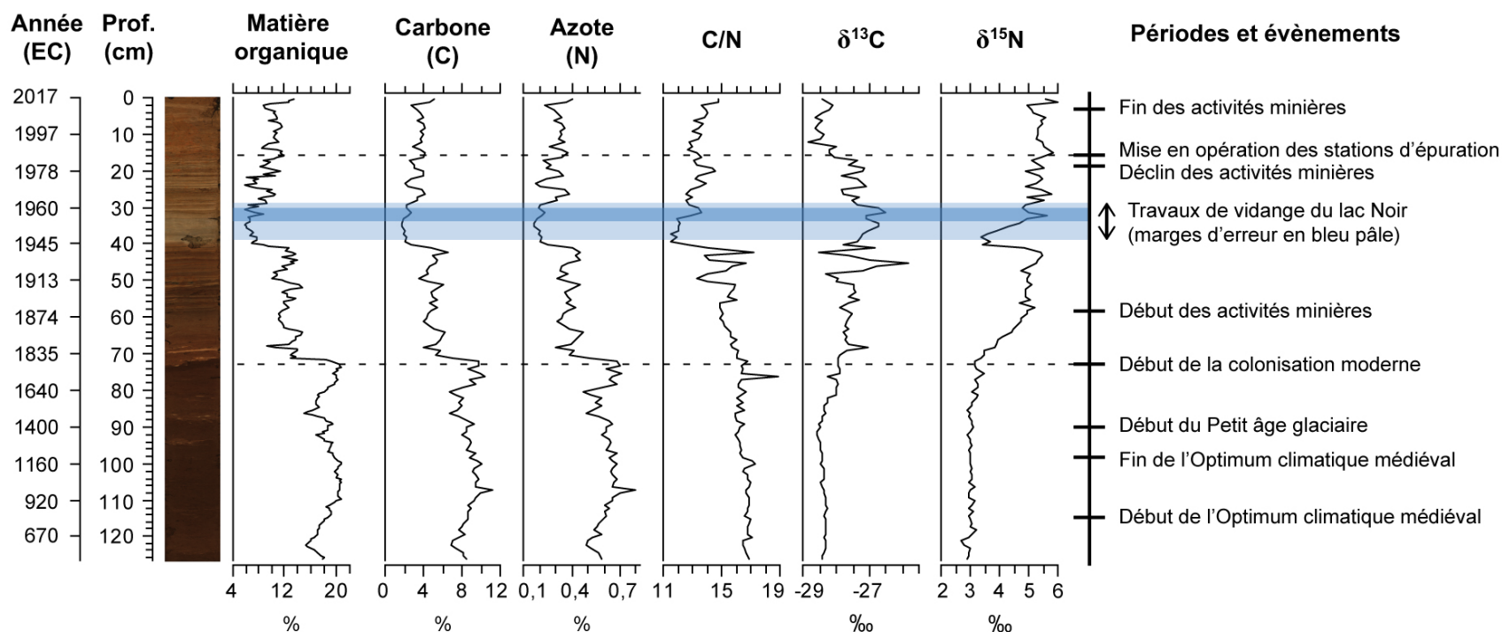
Figure 9.4. Profils de variation des concentrations en matière organique, carbone (C) et azote (N) dans la carotte de sédiments du lac William. Les rapports du carbone sur l'azote (C/N) et des isotopes stables du carbone 13 sur le carbone 12 ( \delta^{13}\text{C} ) et de l'azote 15 sur l'azote 14 ( \delta^{15}\text{N} ) sont également présentés. Note : les traits pointillés marquent le début de la colonisation moderne de la Haute-Bécancour (~ 1810 EC) et la mise en opération des stations d'épuration de Saint-Ferdinand et Thetford Mines (1985–1986 EC).
