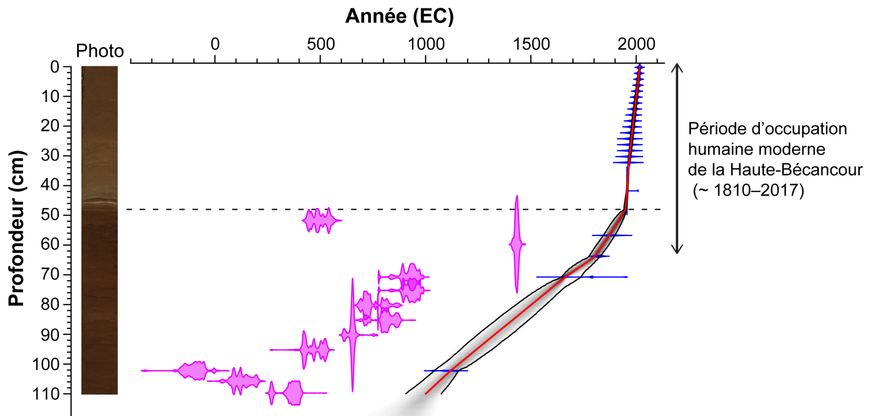
Figure 8.1. Présentation de la carotte de sédiments du lac à la Truite et de son modèle chronologique. Note : la photo illustre l'intérieur de la carotte (plan longitudinal). La ligne rouge représente la courbe d'âge associée aux différents niveaux de profondeurs. Les lignes noires délimitent les intervalles d'erreur (niveau de confiance de 95 %). Les marqueurs bleus désignent les dates qui ont été retenues afin d'établir le modèle, tandis que les marqueurs mauves représentent les dates qui ont été exclues. La ligne pointillée horizontale marque une coupure stratigraphique importante qui a été considérée pour l'élaboration du modèle chronologique.
