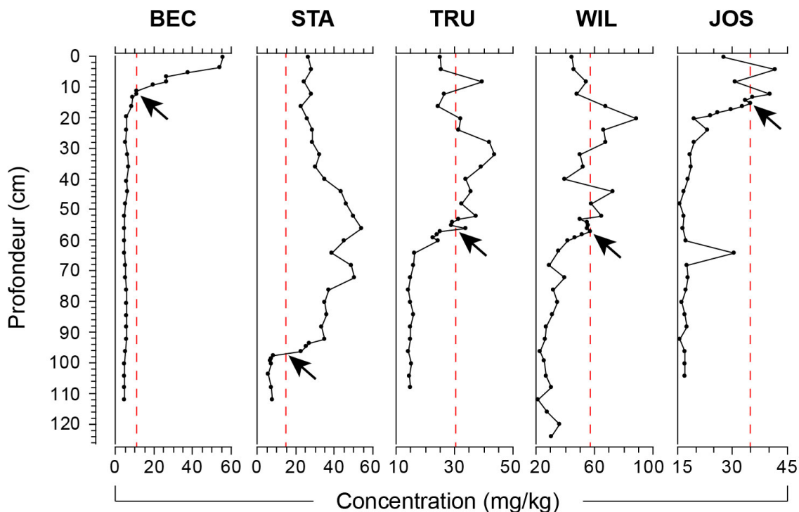
Figure 4.8. Profils de variation de la concentration de plomb stable (Pb) dans les carottes de sédiments du lac Bécancour (BEC), de l'étang Stater (STA), du lac à la Truite (TRU), du lac William (WIL) et du lac Joseph (JOS). Note : les traits pointillés rouges représentent le double de la concentration naturelle de fond de chaque carotte. La date de 1886 \pm 30 EC a été attribuée aux premiers points d'intersection du bas vers le haut entre ces traits et les courbes de concentration (voir flèches).
