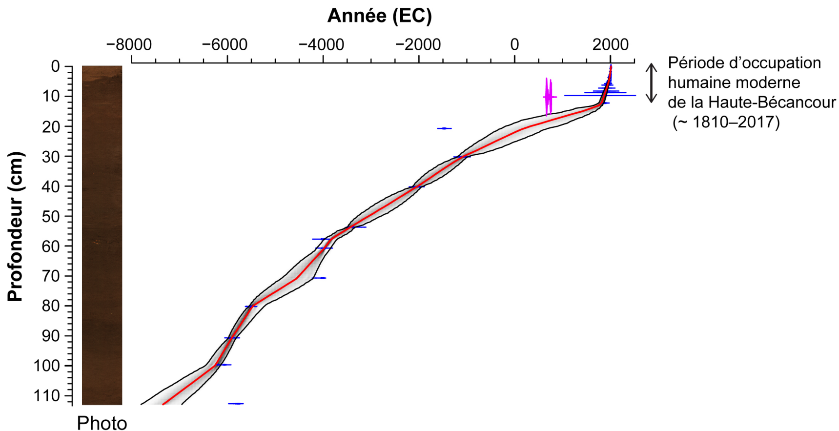
Figure 6.1. Présentation de la carotte de sédiments du lac Bécancour et de son modèle chronologique. Note : la photo illustre l'intérieur de la carotte (plan longitudinal). La ligne rouge représente la courbe d'âge associée aux différents niveaux de profondeurs. Les lignes noires délimitent les intervalles d'erreur (niveau de confiance de 95 %). Les marqueurs bleus désignent les dates qui ont été retenues afin d'établir le modèle, tandis que le marqueur mauve (coin supérieur droit) représente une date qui a été exclue.
