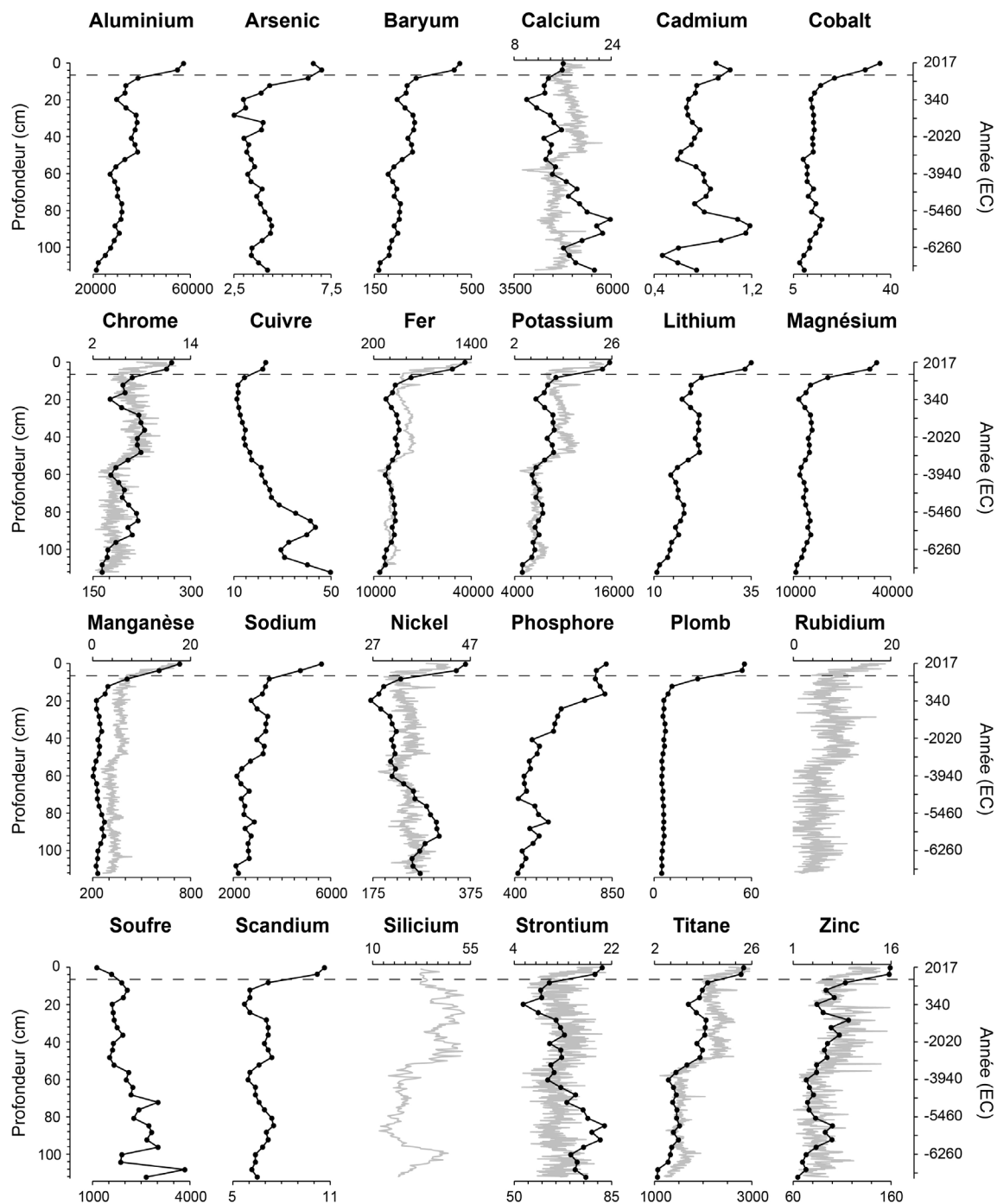
Figure 6.5. Profils de variation de la concentration absolue en métaux et autres éléments chimiques dans la carotte de sédiments du lac Bécancour. Note : les courbes et points noirs (axes horizontaux inférieurs) représentent les données de concentrations (en mg/kg) établies par spectrométrie, tandis que les courbes grises (axes horizontaux supérieurs) correspondent aux données de concentrations relatives obtenues par microfluorescence X. La ligne pointillée marque la construction du barrage vers 1940 EC.
