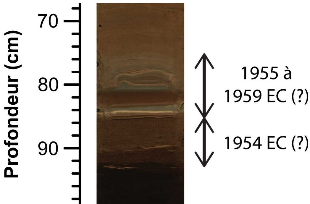
Figure 7.12. Aperçu agrandi des couches de sédiments déposées dans l'étang Stater durant les travaux de vidange du lac Noir (1954–1959 EC). Note : les couches (75 à 93 cm de profondeur) ont été déterminées à partir du modèle chronologique (en considérant les marges d'erreur associées aux dates) et de l'observation de la stratigraphie.
