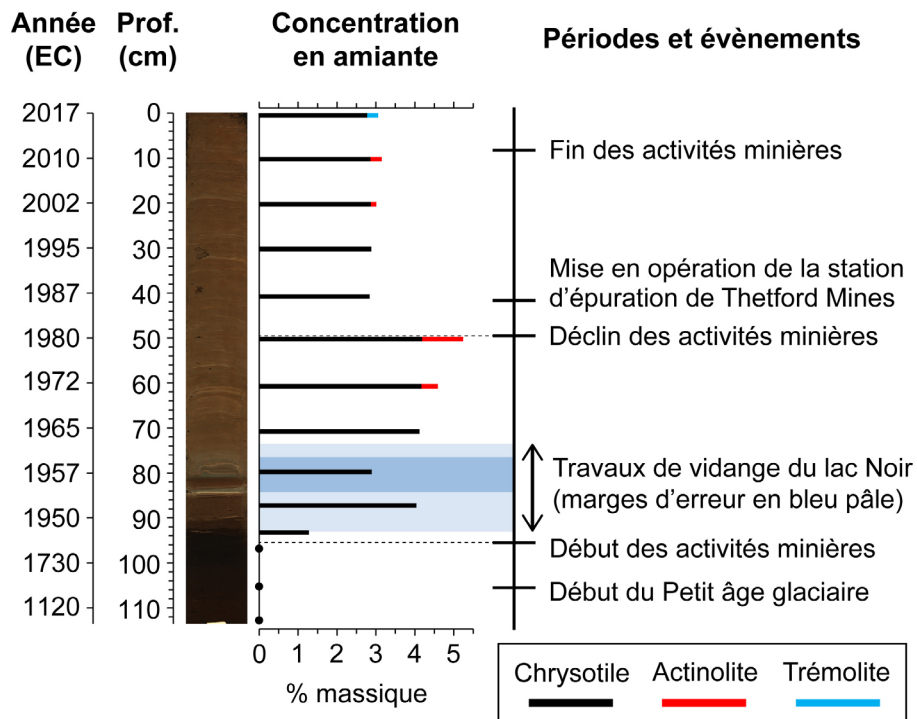
Figure 7.9. Concentration en fibres d'amiante à différents niveaux de profondeur de la carotte de sédiments de l'étang Stater. Note : les traits pointillés marquent le début des activités minières d'amiante dans la Haute-Bécancour (~ 1880 EC) et le début du déclin de l'industrie minière régionale (1980 EC).
