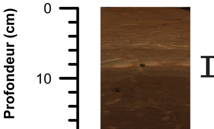
Figure 10.13. Aperçu agrandi des couches de sédiments déposées dans le lac Joseph durant les travaux de vidange du lac Noir (1954–1959 EC). Note : les couches sont délimitées par le marqueur noir (7 à 9,75 cm de profondeur). Elles ont été déterminées à partir du modèle chronologique (en considérant les marges d'erreur associées aux dates) et de l'observation de la stratigraphie.
