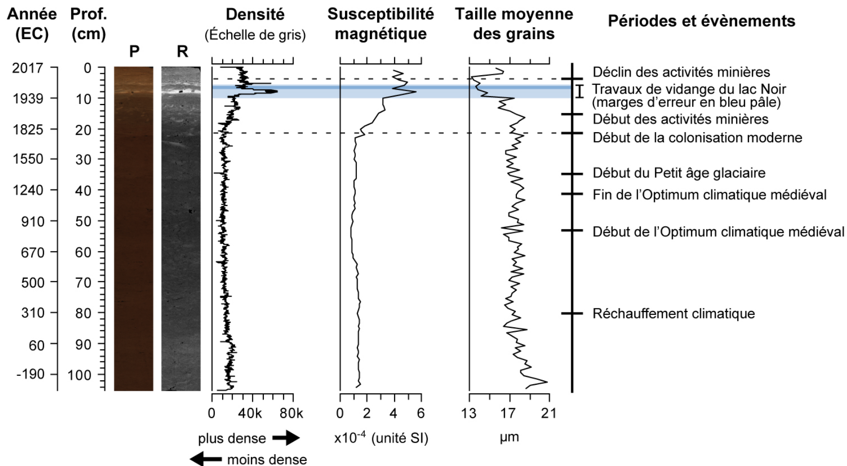
Figure 10.3. Profils de variation de la densité, de la susceptibilité magnétique et de la taille moyenne des grains dans la carotte de sédiments du lac Joseph. Note : les traits pointillés marquent le début de la colonisation moderne de la Haute-Bécancour (~ 1810 EC) et le début du déclin des activités minières d'amiante (1980 EC). P, photographie; R, radiographie.
