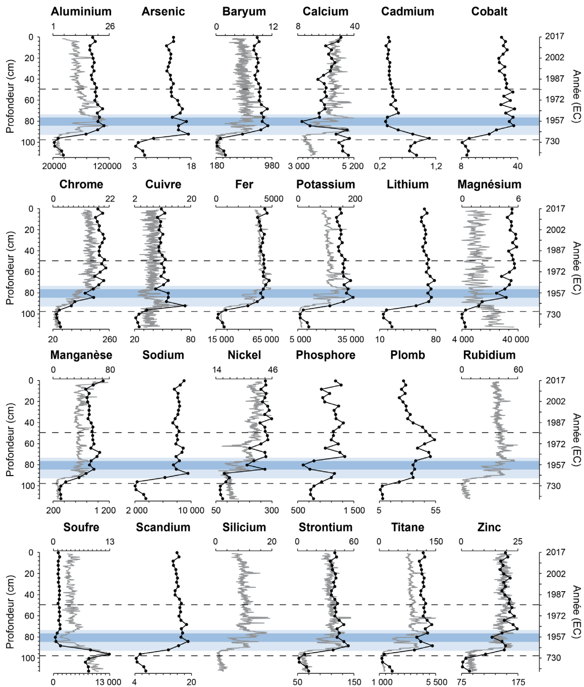
Figure 7.5. Profils de variation de la concentration absolue en métaux et autres éléments chimiques dans la carotte de sédiments de l'étang Stater. Note : les courbes et points noirs (axes horizontaux inférieurs) représentent les données de concentrations (en mg/kg) établies par spectrométrie, tandis que les courbes grises (axes horizontaux supérieurs) correspondent aux données de concentrations relatives obtenues par microfluorescence X. Les zones colorées délimitent la période de travaux de vidange du lac Noir (1954–1959 EC; marges d'erreur en bleu pâle), tandis que les traits pointillés inférieur et supérieur marquent respectivement le début de la colonisation moderne de la Haute-Bécancour (~ 1810 EC) et le début du déclin des activités minières d'amiante (1980 EC).
