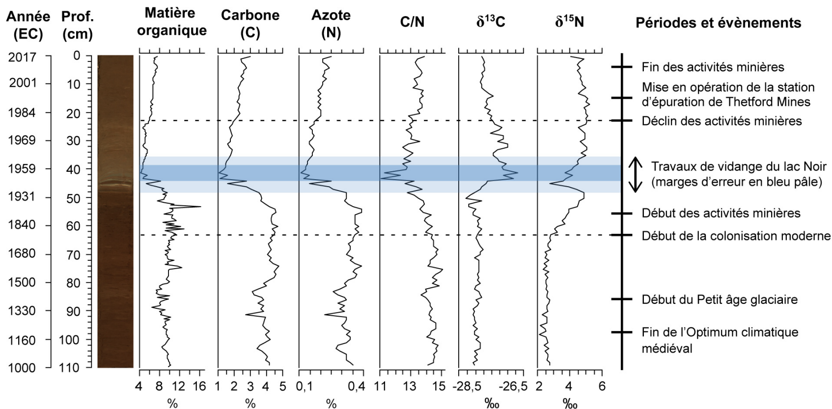
Figure 8.4. Profils de variation des concentrations en matière organique, carbone (C) et azote (N) dans la carotte de sédiments du lac à la Truite. Les rapports du carbone sur l'azote (C/N) et des isotopes stables du carbone 13 sur le carbone 12 ( \delta^{13}\text{C} ) et de l'azote 15 sur l'azote 14 ( \delta^{15}\text{N} ) sont également présentés. Note : les traits pointillés marquent le début de la colonisation moderne de la Haute-Bécancour (~ 1810 EC) et le début du déclin des activités minières d'amiante (1980 EC).
